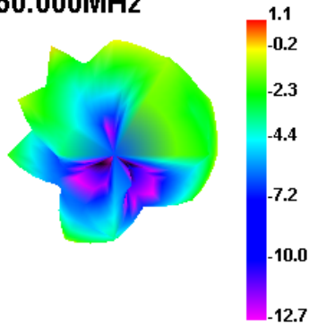
5650.000MHz E1
