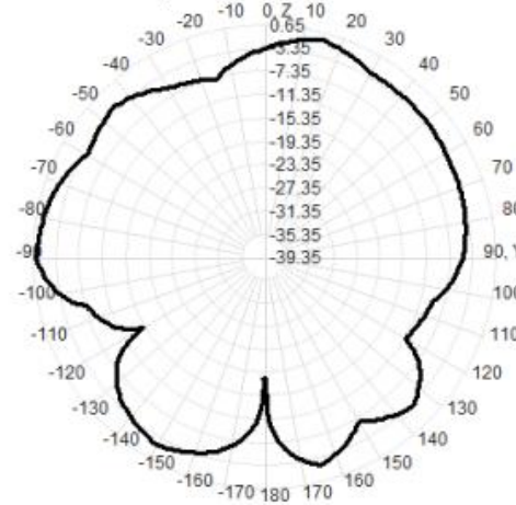
2400.0MHz Total(E2-YZ), Max= -0.01dBi
