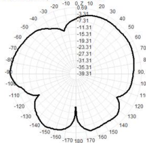
2500.0MHz Total(E2-YZ), Max= 0.41dBi
