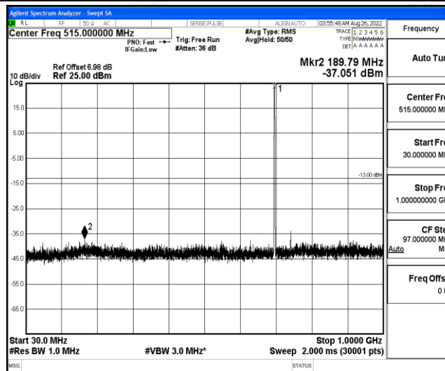
Band12-10MHz-QPSK-23095-1-0-Low-30-1000--37.05-PASS
