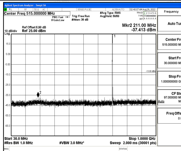
Band12-1.4MHz-16QAM-23095-1-0-Low-30-1000--37.41-PASS
