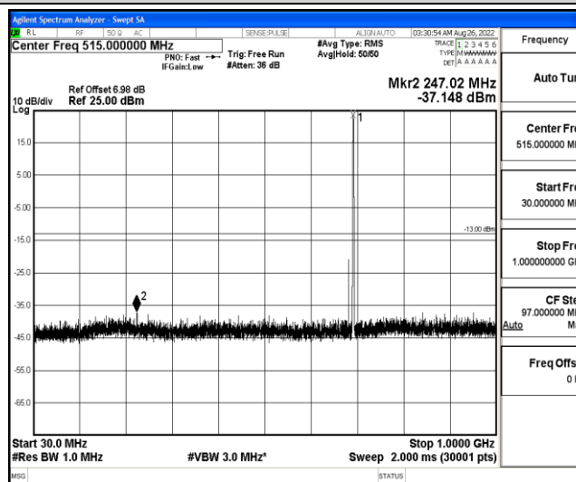
Band12-5MHz-QPSK-23035-1-0-Low-30-1000--37.15-PASS
