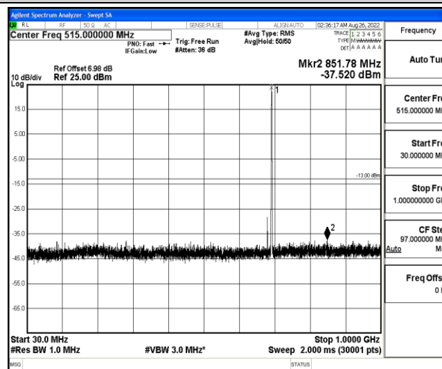
Band12-1.4MHz-16QAM-23017-1-0-Low-30-1000--37.52-PASS
