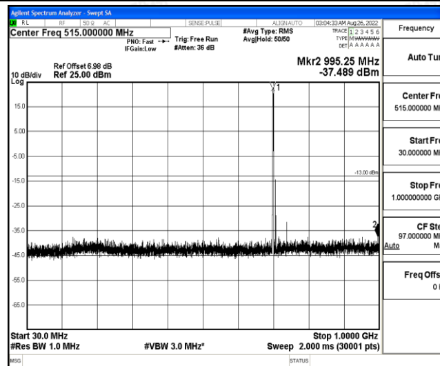
Band12-3MHz-QPSK-23095-1-0-Low-30-1000--37.49-PASS
