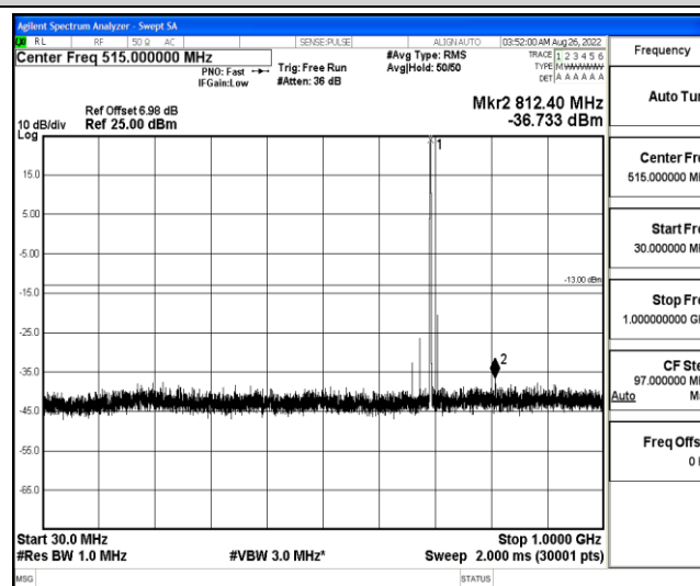
Band12-10MHz-QPSK-23060-1-0-Low-30-1000--36.73-PASS
