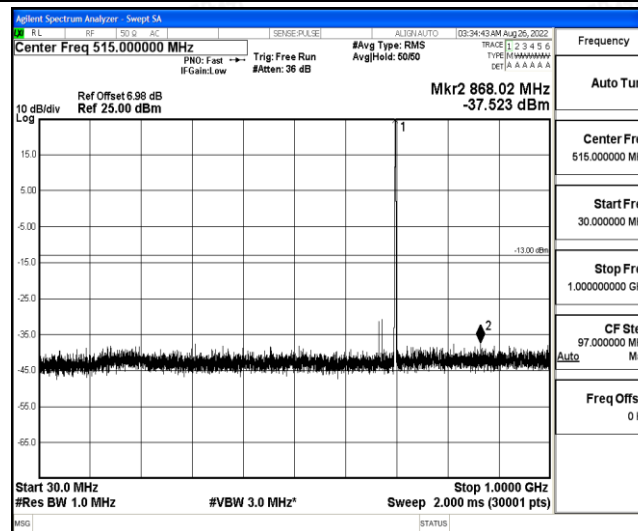
Band12-5MHz-QPSK-23095-1-0-Low-30-1000--37.52-PASS
