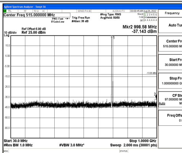
Band12-3MHz-QPSK-23025-1-0-Low-30-1000--37.14-PASS
