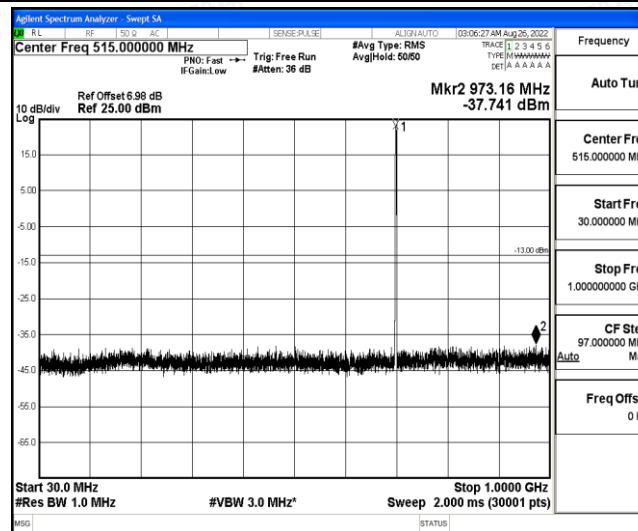
Band12-3MHz-16QAM-23095-1-0-Low-30-1000--37.74-PASS
