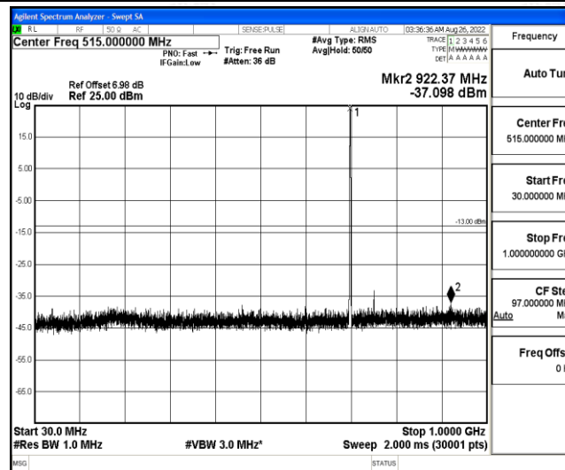
Band12-5MHz-16QAM-23095-1-0-Low-30-1000--37.1-PASS
