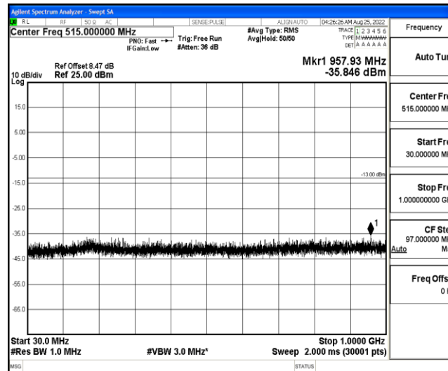
Band4-20MHz-QPSK-20050-1-0-Low-30-1000--35.85-PASS
