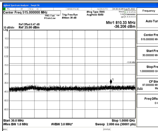
Band4-20MHz-QPSK-20175-1-0-Low-30-1000--36.21-PASS
