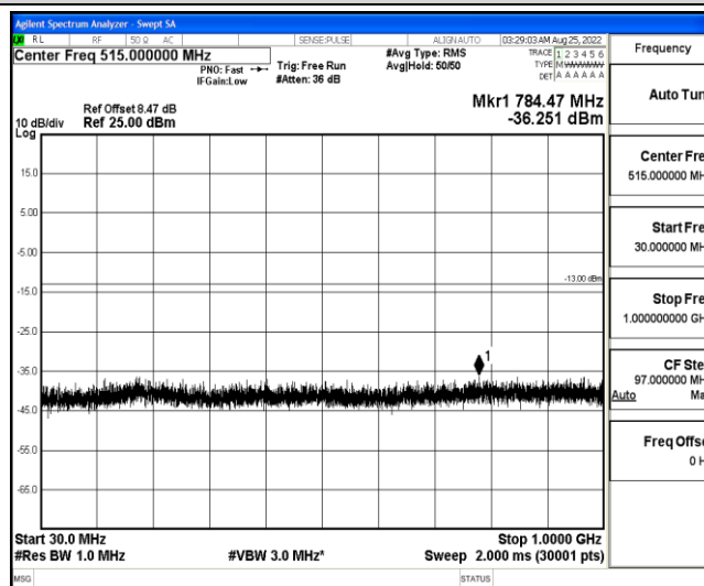
Band4-5MHz-QPSK-20175-1-0-Low-30-1000--36.25-PASS
