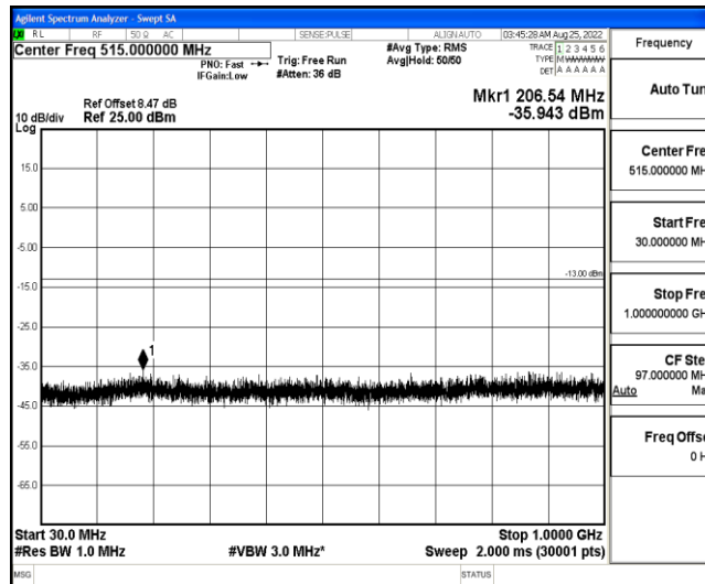
Band4-10MHz-QPSK-20000-1-0-Low-30-1000--35.94-PASS
