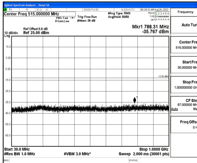
Band2-20MHz-QPSK-18700-1-0-Low-30-1000--35.77-PASS
