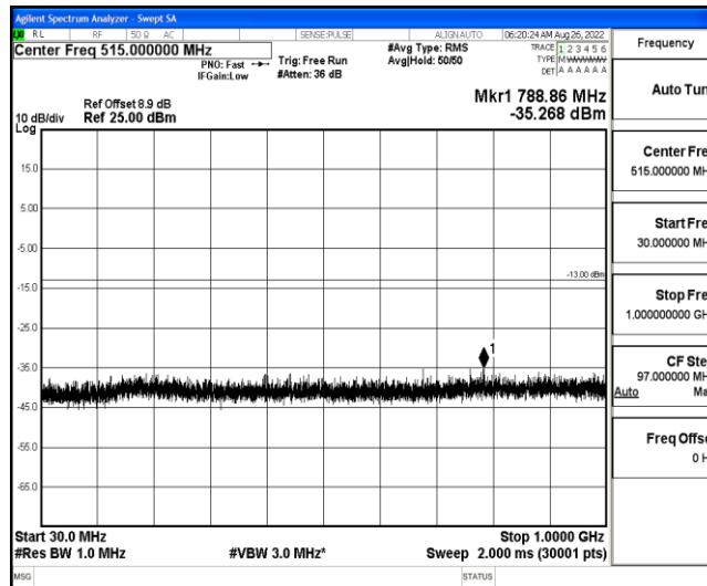
Band2-20MHz-16QAM-18700-1-0-Low-30-1000--35.27-PASS
