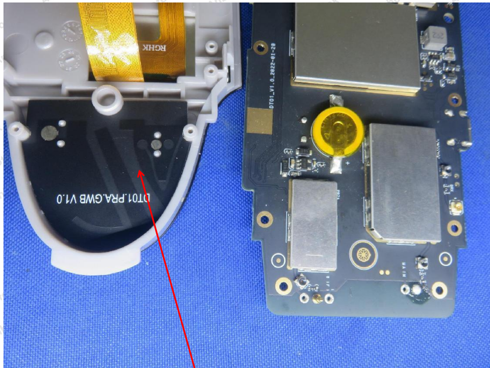
BT/WIFI/GPS(RX) ANT
