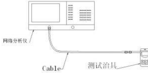
测试示意图
