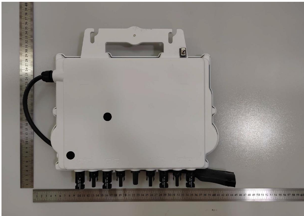
8) EUT Photo
