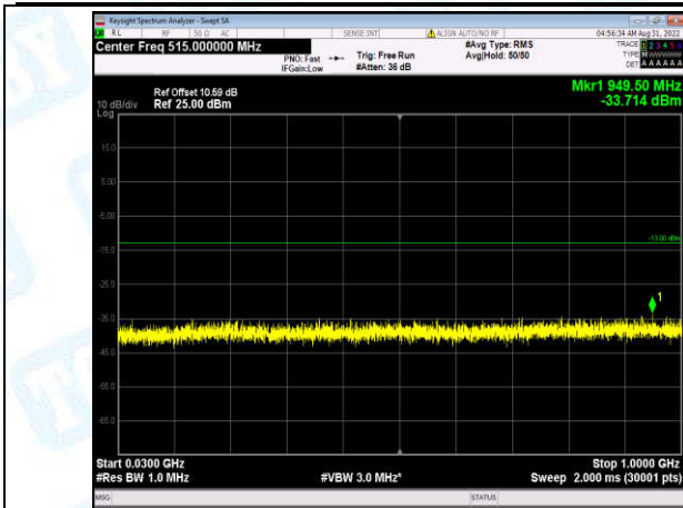
Band2-20MHz-QPSK-18900-1-0-Low-30-1000--33.71-PASS
