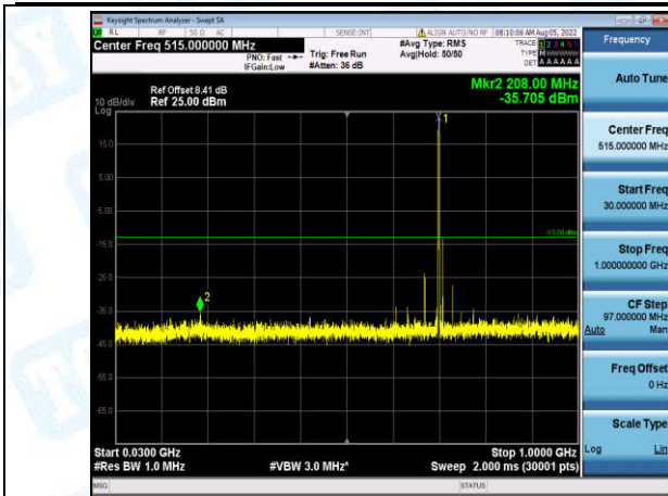
Band12-3MHz-16QAM-23095-1-0-Low-30-1000--35.71-PASS
