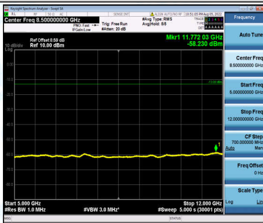
Band13-5MHz-QPSK-23230-1-0-Low-5000-12000--58.23-PASS
