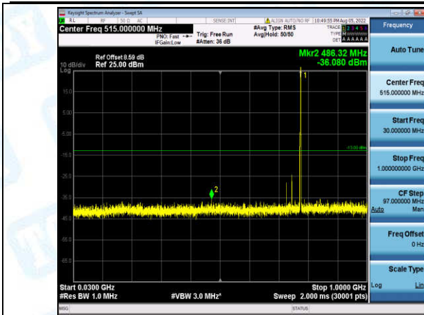
Band13-5MHz-QPSK-23230-1-0-Low-30-1000--36.08-PASS
