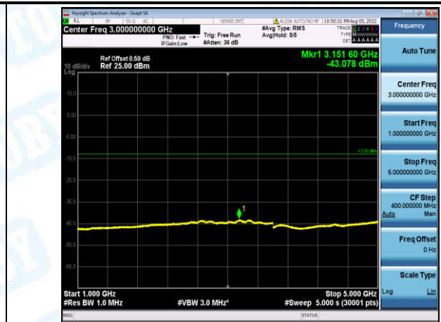
Band13-5MHz-QPSK-23230-1-0-Low-1000-5000--43.08-PASS
