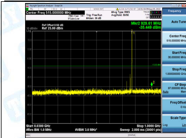
Band13-5MHz-16QAM-23230-1-0-Low-30-1000--35.45-PASS
