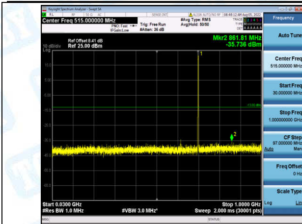
Band12-5MHz-QPSK-23095-1-0-Low-30-1000--35.74-PASS
