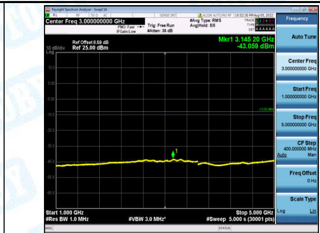
Band13-5MHz-16QAM-23230-1-0-Low-1000-5000--43.06-PASS
