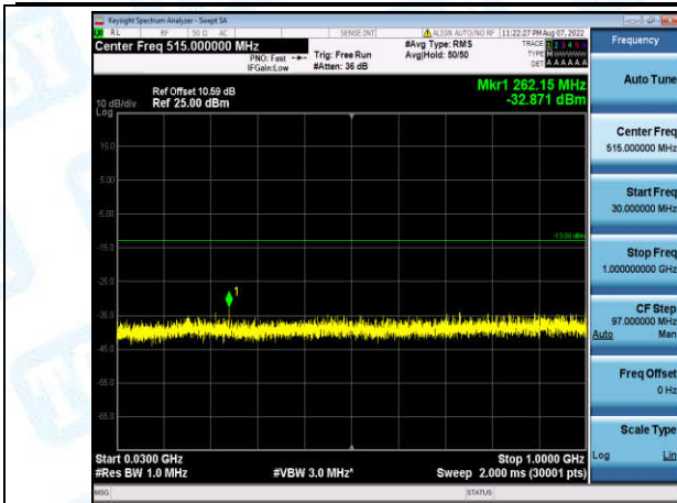
Band2-3MHz-QPSK-18900-1-0-Low-30-1000--32.87-PASS
