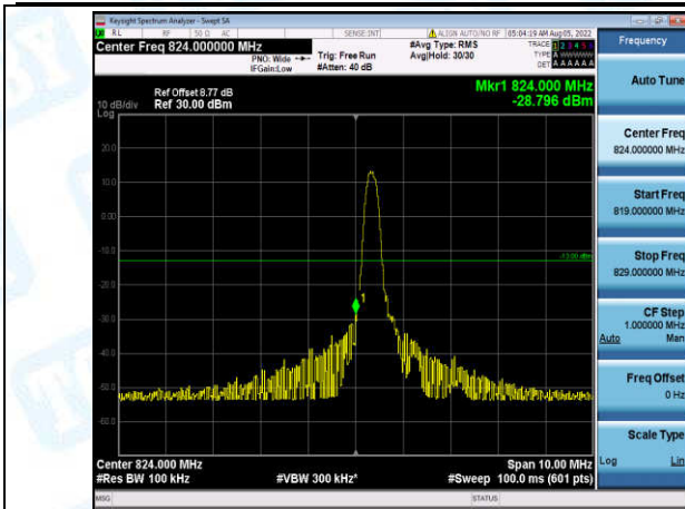
Band5-5MHz-16QAM-20425-1-0-Low--28.80-PASS
