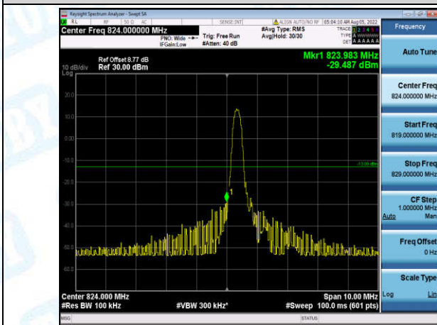
Band5-5MHz-QPSK-20425-1-0-Low--29.49-PASS
