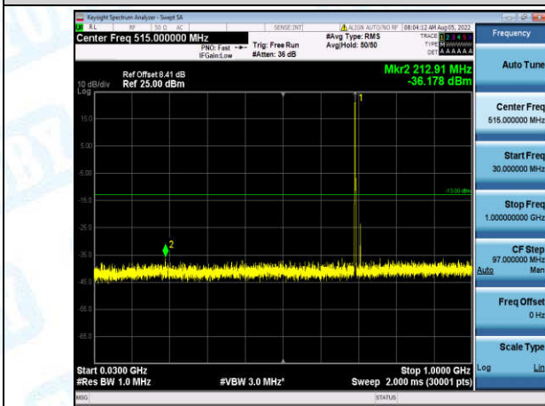
Band12-3MHz-QPSK-23025-1-0-Low-30-1000--36.18-PASS
