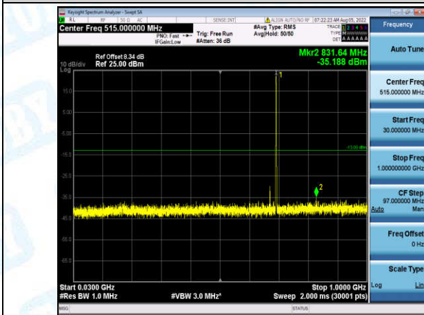
Band12-1.4MHz-16QAM-23017-1-0-Low-30-1000--35.19-PASS
