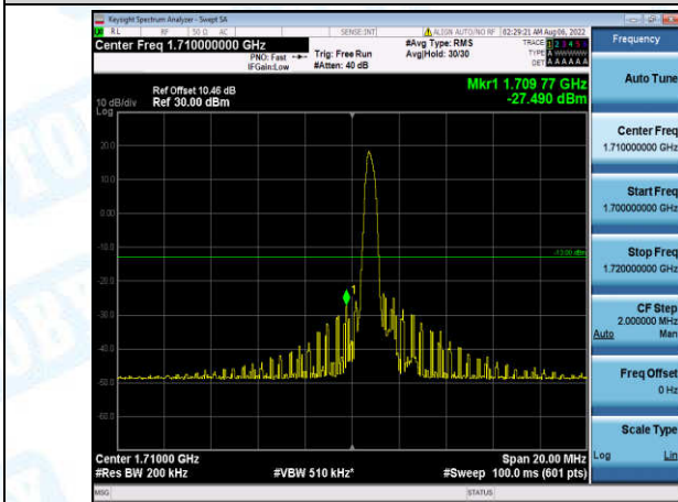
Band4-10MHz-QPSK-20000-1-0-Low--27.49-PASS
