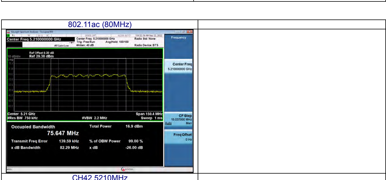
CH42 5210MHz
