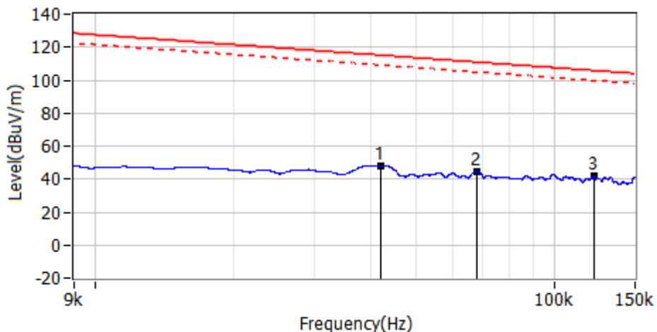
9KHz-150KHz
