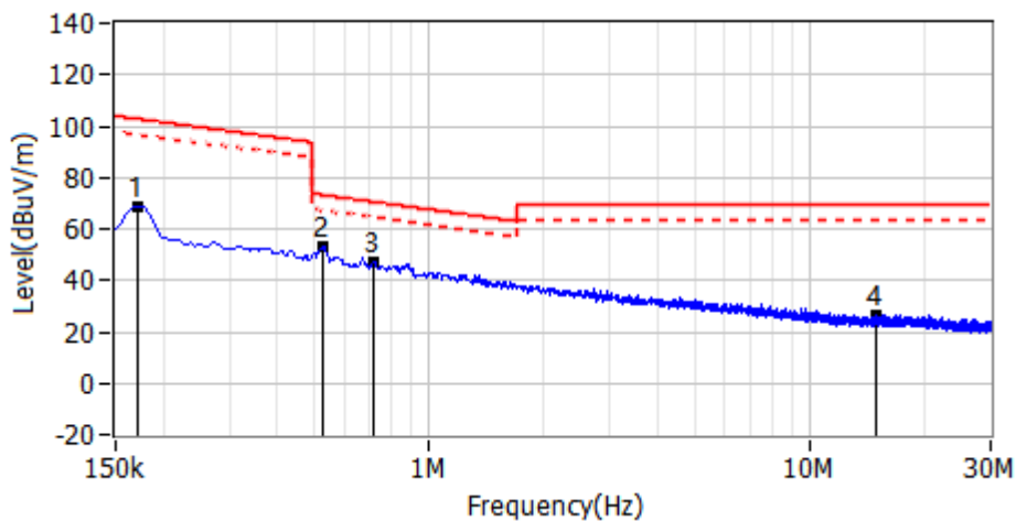
150KHz-30MHz
