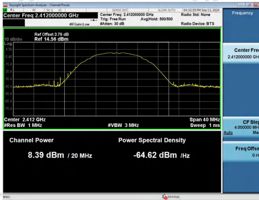
MAX__Output_Power_NVNT_ANT1_802_11b_2412
