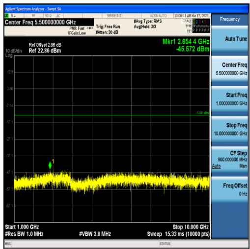
Band71-10MHz-QPSK-133297-50RB#0-Range2:1000~10000MHz
