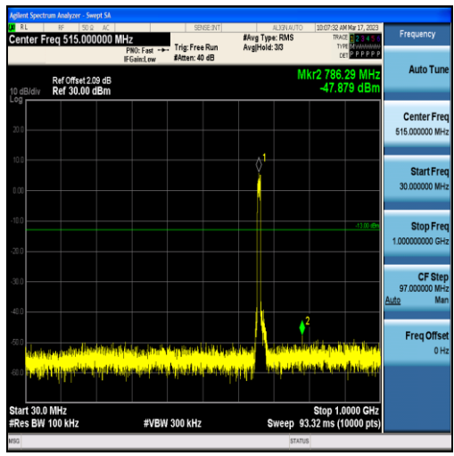
Band71-10MHz-QPSK-133172-50RB#0-Range1:30~1000MHz
