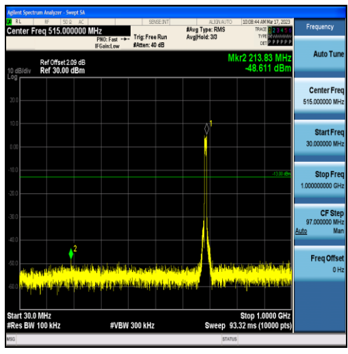
Band71-10MHz-QPSK-133422-50RB#0-Range1:30~1000MHz
