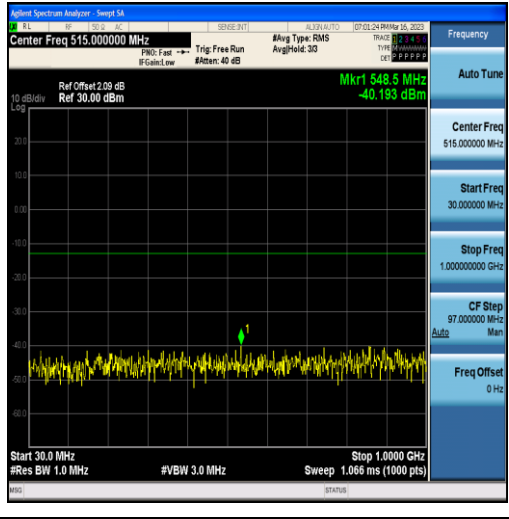
Band25-10MHz-QPSK-26365-50RB#0-Range1:30~1000MHz
