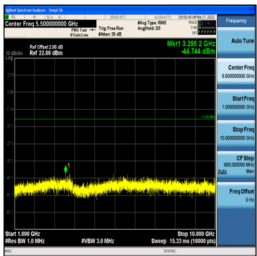
Band71-5MHz-QPSK-133147-25RB#0-Range2:100~10000MHz
