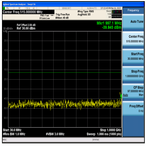
Band25-20MHz-QPSK-26365-100RB#0-Range1:30~1000MHz
