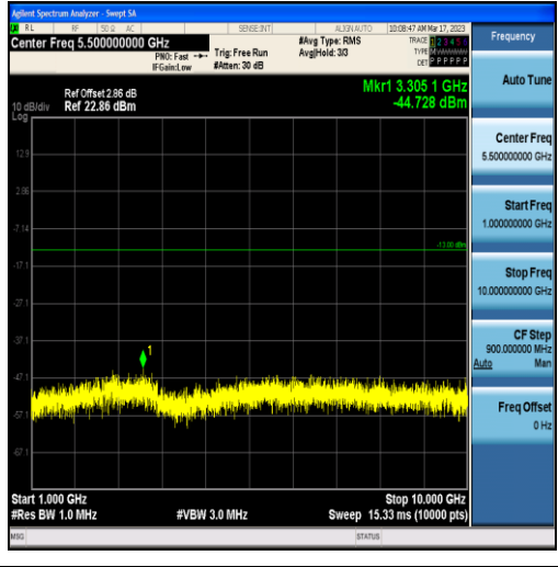
Band71-10MHz-QPSK-133422-50RB#0-Range2:1000~10000MHz
