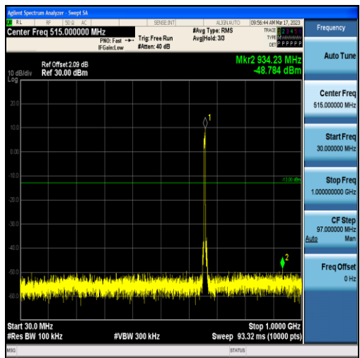
Band71-5MHz-QPSK-133147-25RB#0-Range1:30~1000MHz
