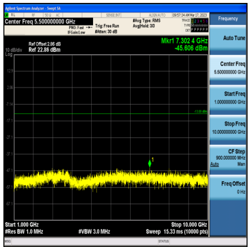
Band71-5MHz-QPSK-133447-25RB#0-Range2:1000~10000MHz
