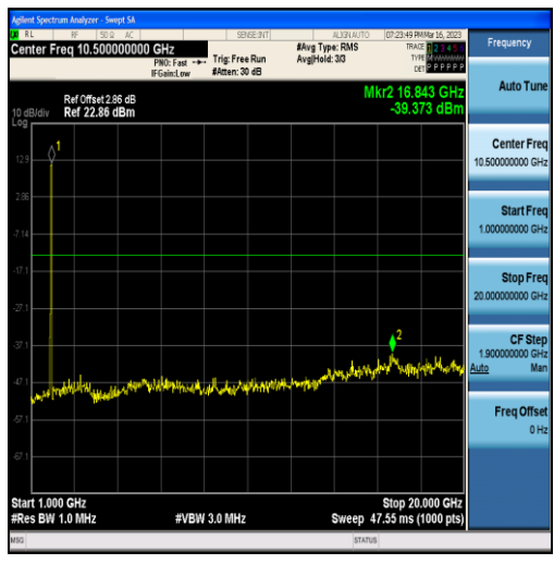
Band25-20MHz-QPSK-26365-100RB#0-Range2:1000~20000MHz
