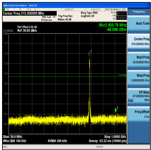
Band71-5MHz-QPSK-133447-25RB#0-Range1:30~1000MHz
