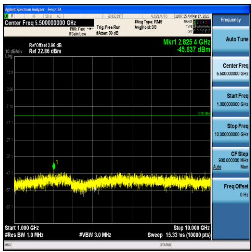
Band71-10MHz-QPSK-133172-50RB#0-Range2:1000~10000MHz
