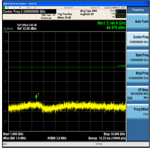
Band71-15MHz-QPSK-133397-75RB#0-Range2:1000~10000MHz
