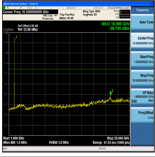
Band25-10MHz-QPSK-26640-50RB#0-Range2:1000~20000MHz
