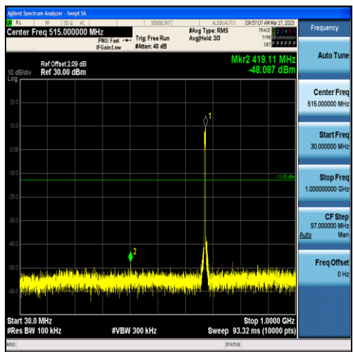
Band71-5MHz-QPSK-133297-25RB#0-Range1:30~1000MHz
