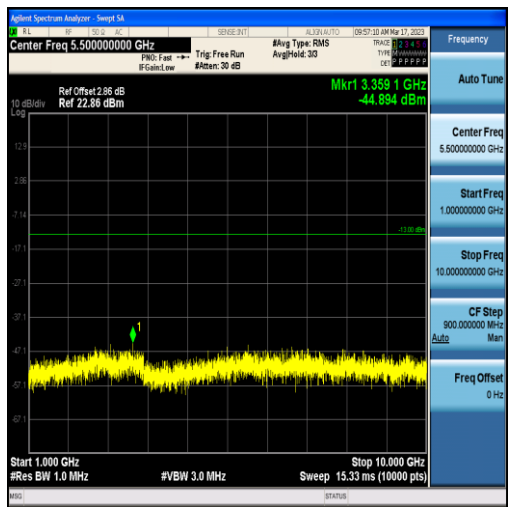
Band71-5MHz-QPSK-133297-25RB#0-Range2:1000~10000MHz
