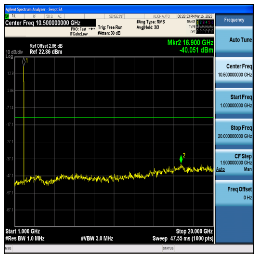
Band25-3MHz-QPSK-26365-15RB#0-Range2:1000~20000MHz
