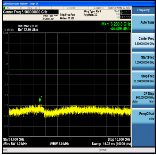
Band17-10MHz-QPSK-23800-50RB#0-Range2:1000~10000MHz
