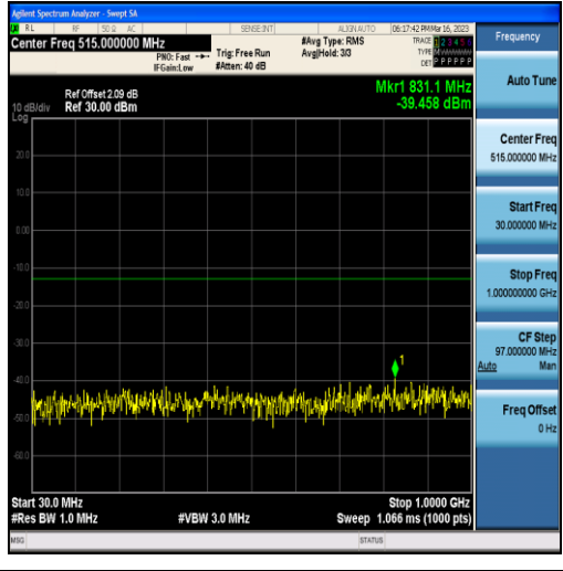
Band25-1.4MHz-QPSK-26047-6RB#0-Range1:30~1000MHz
