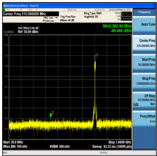
Band12-10MHz-QPSK-23130-50RB#0-Range1:30~1000MHz
