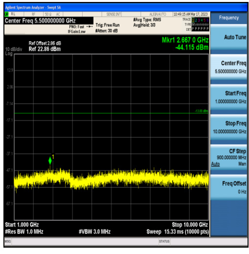
Band13-5MHz-QPSK-23255-25RB#0-Range2:1000~10000MHz
