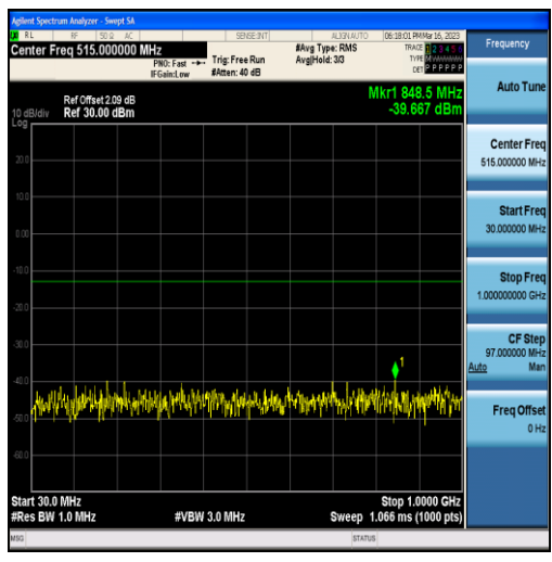
Band25-1.4MHz-QPSK-26365-6RB#0-Range1:30~1000MHz
