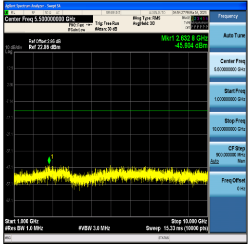
Band12-10MHz-QPSK-23130-50RB#0-Range2:1000~10000MHz
