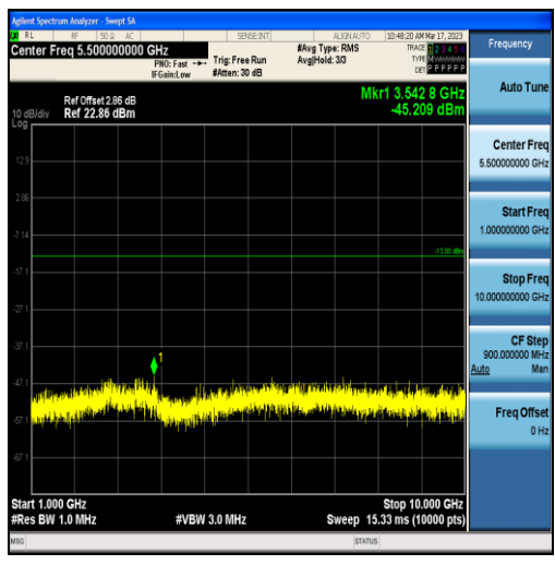
Band13-5MHz-QPSK-23205-25RB#0-Range2:1000~10000MHz
