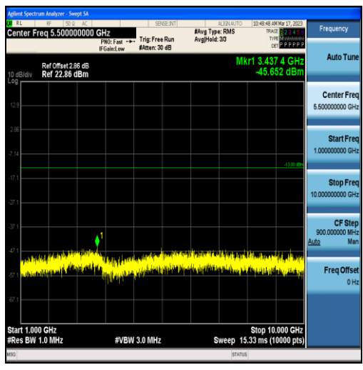
Band13-5MHz-QPSK-23230-25RB#0-Range2:1000~10000MHz
