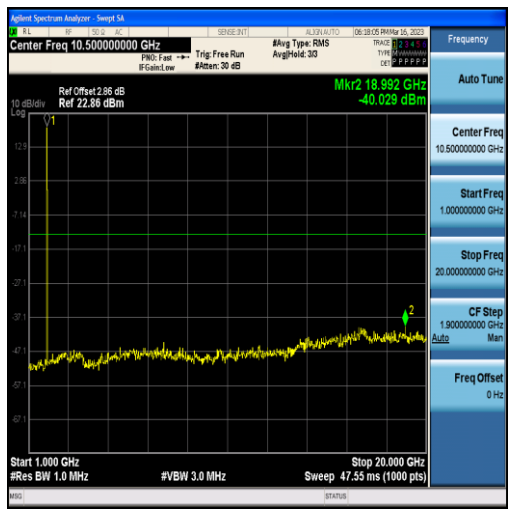
Band25-1.4MHz-QPSK-26365-6RB#0-Range2:1000~20000MHz
