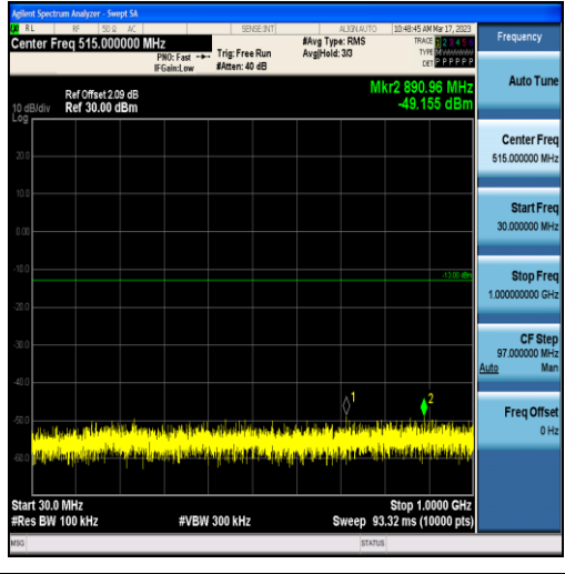
Band13-5MHz-QPSK-23230-25RB#0-Range1:30~1000MHz
