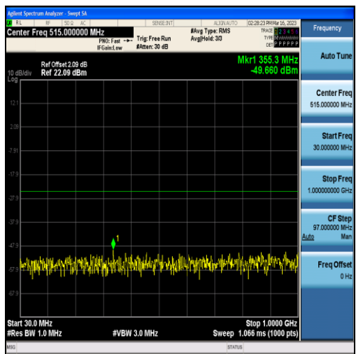
Band7-20MHz-QPSK-20850-100RB#0-Range1:30~1000MHz
