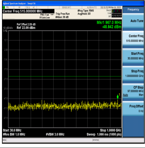
Band7-20MHz-QPSK-21350-100RB#0-Range1:30~1000MHz
