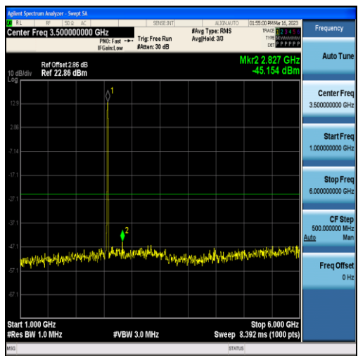
Band7-10MHz-QPSK-21400-50RB#0-Range2:1000~6000MHz
