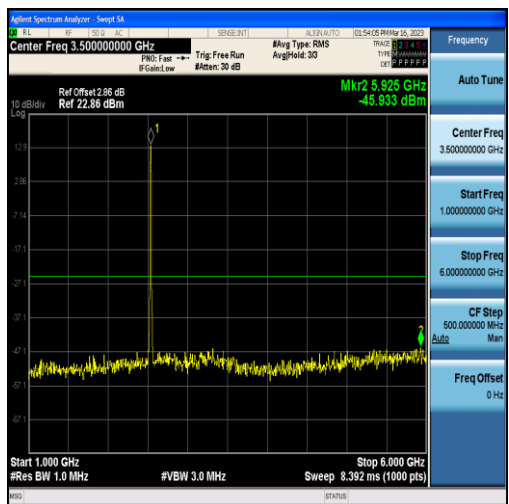
Band7-10MHz-QPSK-21100-50RB#0-Range2:1000~6000MHz
