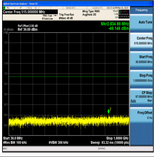
Band12-1.4MHz-QPSK-23017-6RB#0-Range1:30~1000MHz
