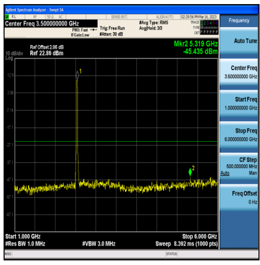
Band7-20MHz-QPSK-21100-100RB#0-Range2:1000~6000MHz
