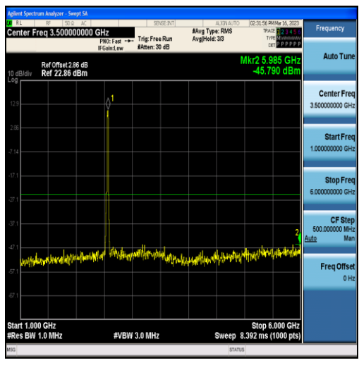
Band7-20MHz-QPSK-21350-100RB#0-Range2:1000~6000MHz
