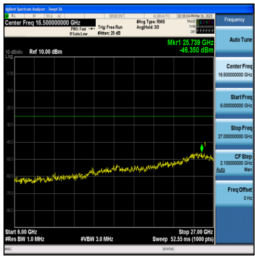
Band7-20MHz-QPSK-21100-100RB#0-Range3:6000~27000MHz
