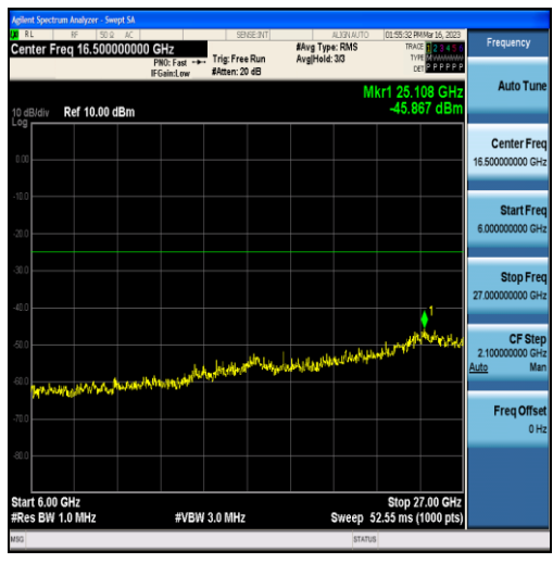
Band7-10MHz-16QAM-21400-50RB#0-Range3:6000~27000MHz
