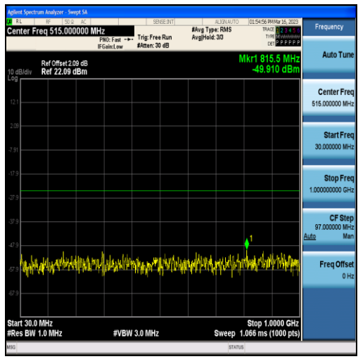
Band7-10MHz-QPSK-21400-50RB#0-Range1:30~1000MHz
