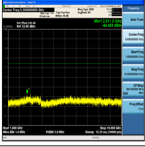
Band12-1.4MHz-QPSK-23017-6RB#0-Range2:1000~10000MHz
