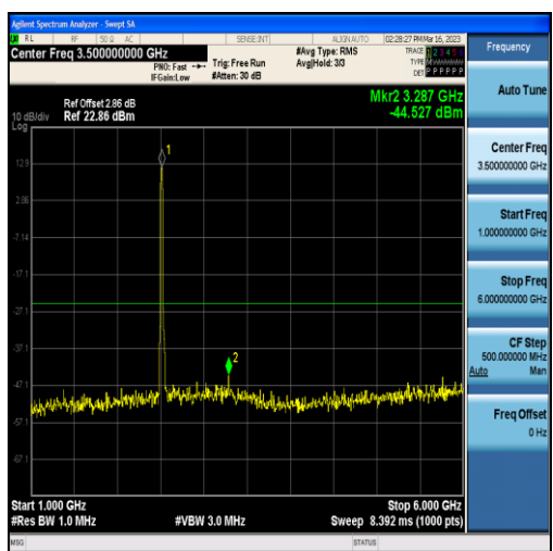
Band7-20MHz-QPSK-20850-100RB#0-Range2:1000~6000MHz
