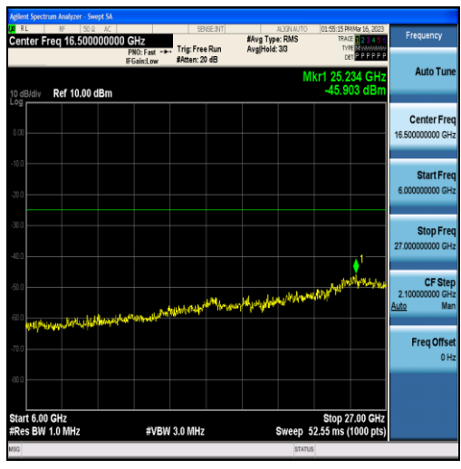
Band7-10MHz-QPSK-21400-50RB#0-Range3:6000~27000MHz
