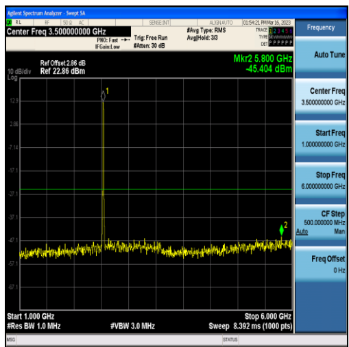
Band7-10MHz-16QAM-21100-50RB#0-Range2:1000~6000MHz
