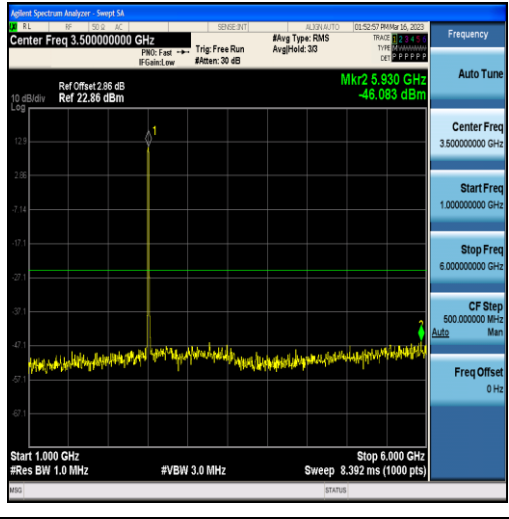
Band7-10MHz-16QAM-20800-50RB#0-Range2:1000~6000MHz
