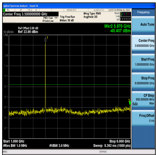
Band7-5MHz-QPSK-20775-25RB#0-Range2:1000~6000MHz
