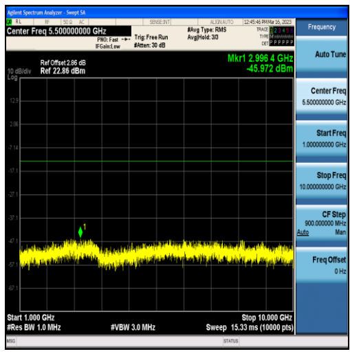
Band5-10MHz-QPSK-20525-50RB#0-Range2:1000~10000MHz
