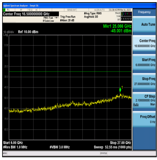
Band7-5MHz-QPSK-21425-25RB#0-Range3:6000~27000MHz
