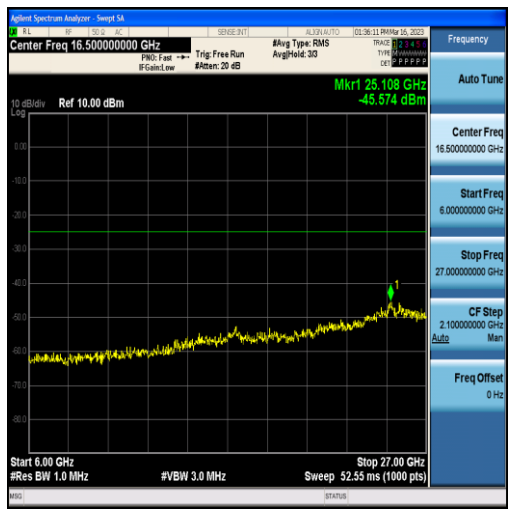
Band7-5MHz-QPSK-20775-25RB#0-Range3:6000~27000MHz
