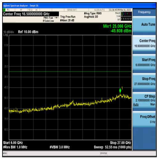
Band7-5MHz-QPSK-21100-25RB#0-Range3:6000~27000MHz
