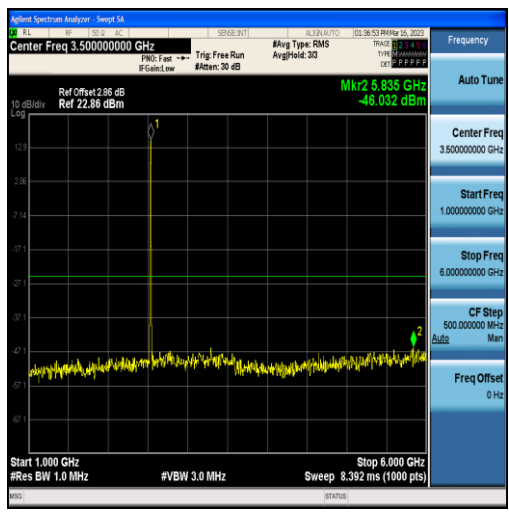
Band7-5MHz-16QAM-21100-25RB#0-Range2:1000~6000MHz
