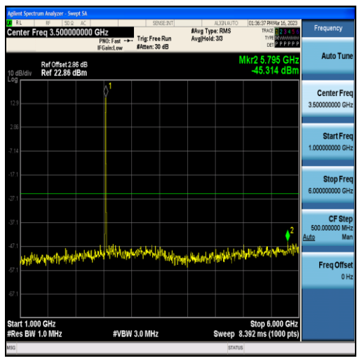
Band7-5MHz-QPSK-21100-25RB#0-Range2:1000~6000MHz
