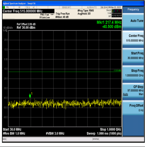
Band4-1.4MHz-QPSK-19957-6RB#0-Range1:30~1000MHz
