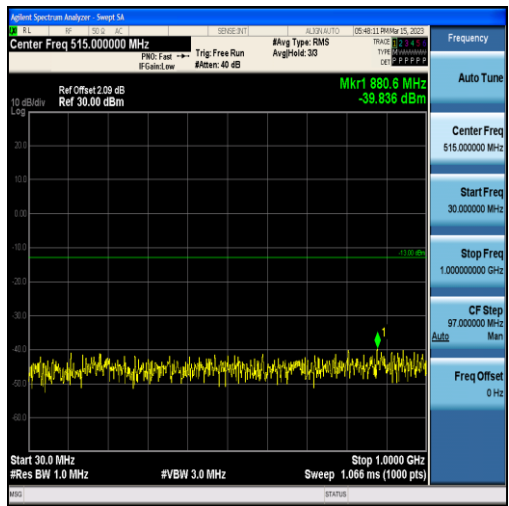
Band2-20MHz-QPSK-18700-100RB#0-Range1:30~1000MHz
