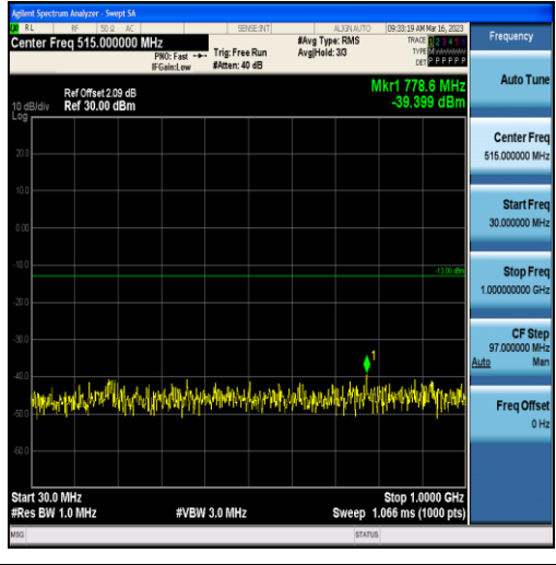
Band4-3MHz-QPSK-19965-15RB#0-Range1:30~1000MHz
