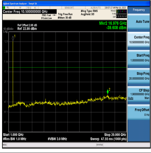
Band4-10MHz-16QAM-20000-50RB#0-Range2:1000~20000MHz
