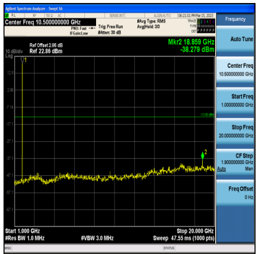
Band4-1.4MHz-QPSK-20393-6RB#0-Range2:1000~20000MHz
