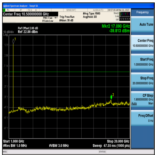
Band4-10MHz-QPSK-20000-50RB#0-Range2:1000~20000MHz
