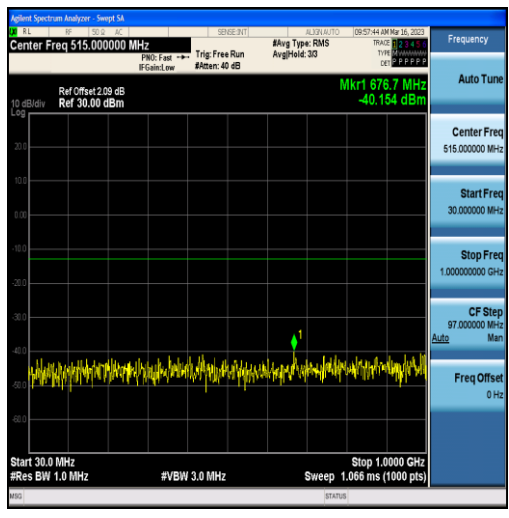
Band4-10MHz-QPSK-20350-50RB#0-Range1:30~1000MHz
