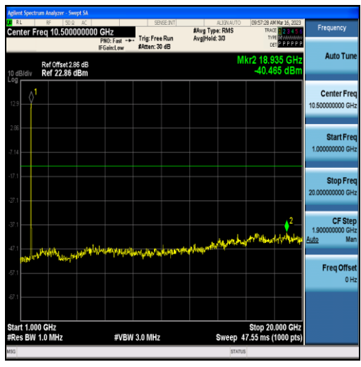
Band4-10MHz-QPSK-20175-50RB#0-Range2:1000~20000MHz
