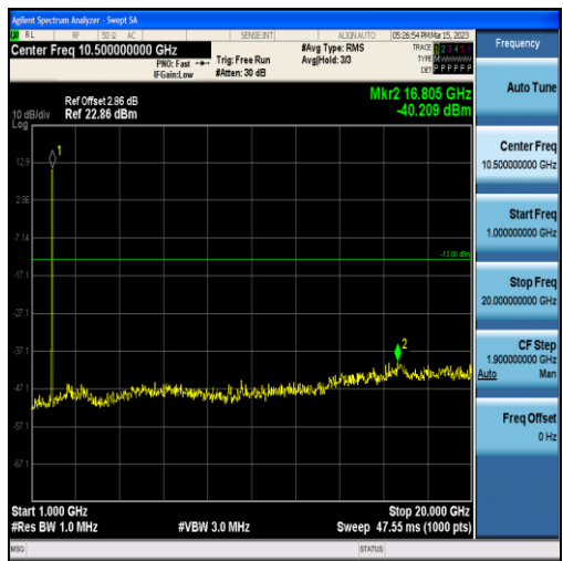
Band2-10MHz-QPSK-18900-50RB#0-Range2:1000~20000MHz
