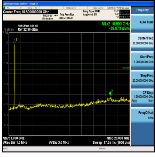
Band2-20MHz-QPSK-19100-100RB#0-Range2:1000~20000MHz
