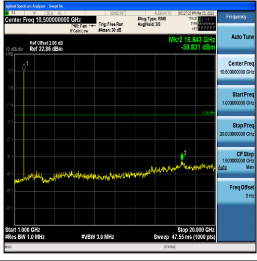
Band2-10MHz-QPSK-19150-50RB#0-Range2:1000~20000MHz
