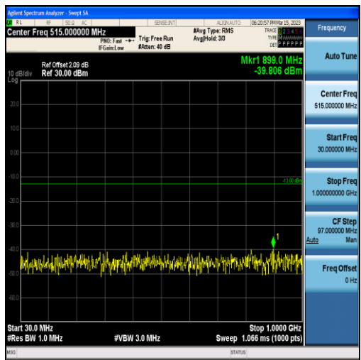
Band4-1.4MHz-QPSK-20393-6RB#0-Range1:30~1000MHz
