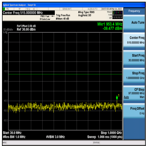
Band4-10MHz-QPSK-20000-50RB#0-Range1:30~1000MHz
