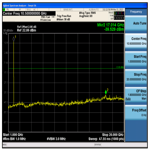
Band2-5MHz-16QAM-18900-25RB#0-Range2:1000~20000MHz
