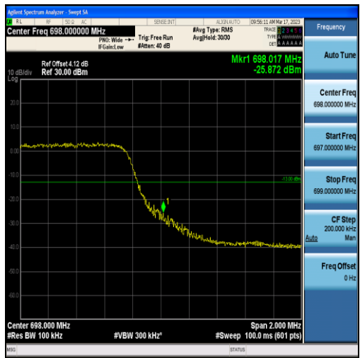
Band71-5MHz-QPSK-133447-25RB#0
