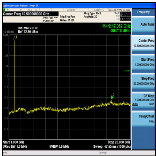
Band2-3MHz-QPSK-18900-15RB#0-Range2:1000~20000MHz
