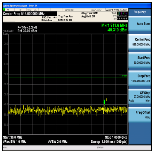
Band2-5MHz-QPSK-18900-25RB#0-Range1:30~1000MHz
