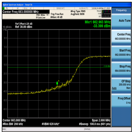
Band71-10MHz-QPSK-133172-50RB#0
