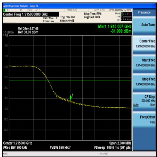
Band25-10MHz-QPSK-26640-50RB#0
