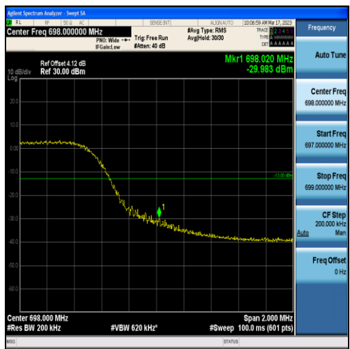
Band71-10MHz-QPSK-133422-50RB#0
