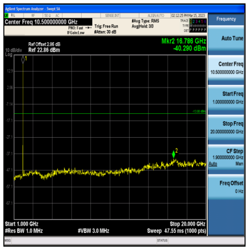
Band2-3MHz-16QAM-19185-15RB#0-Range2:1000~20000MHz
