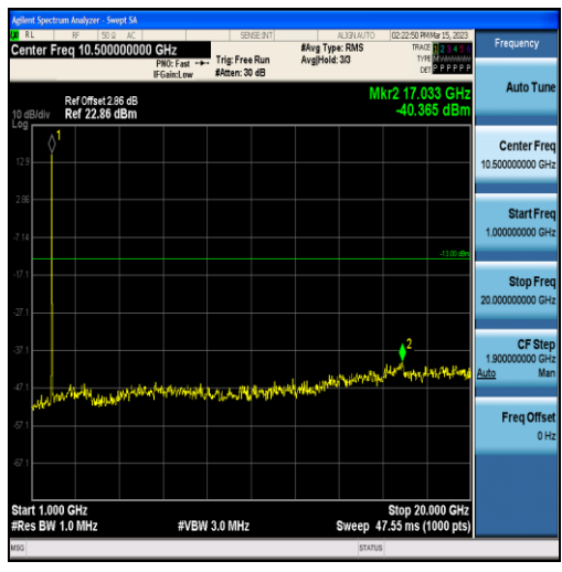
Band2-5MHz-QPSK-18900-25RB#0-Range2:1000~20000MHz
