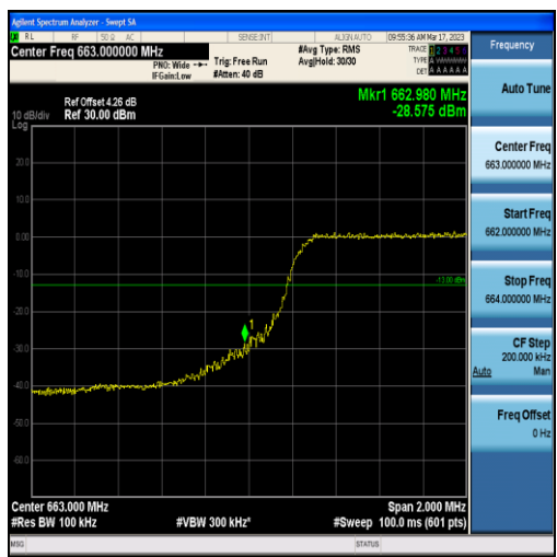
Band71-5MHz-QPSK-133147-25RB#0
