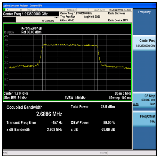
Band25-3MHz-QPSK-26675-15RB#0-2.6886
