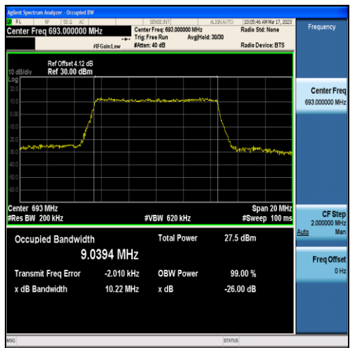
Band71-10MHz-QPSK-133422-50RB#0-9.0394
