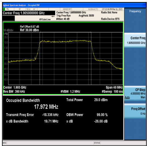
Band25-20MHz-QPSK-26590-100RB#0-17.972
