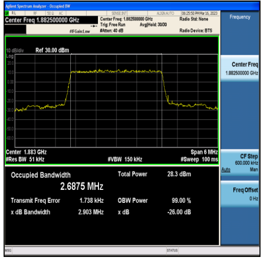
Band25-3MHz-QPSK-26365-15RB#0-2.6875
