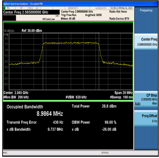
Band7-10MHz-QPSK-21400-50RB#0-8.9864
