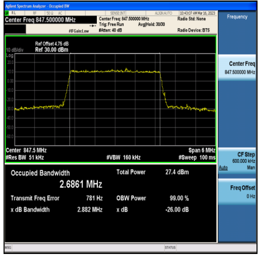
Band5-3MHz-QPSK-20635-15RB#0-2.6861
