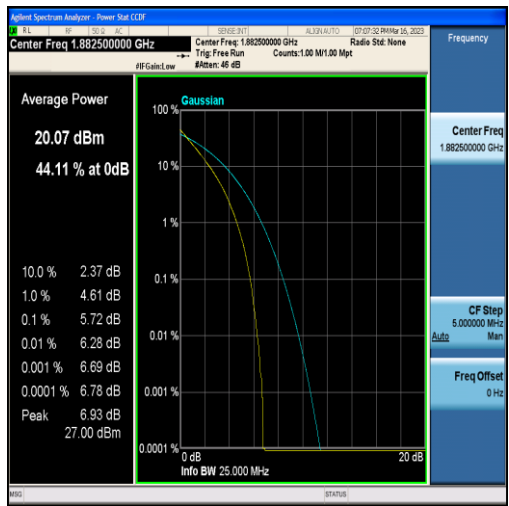
Band25-10MHz-QPSK-26365-50RB#0
