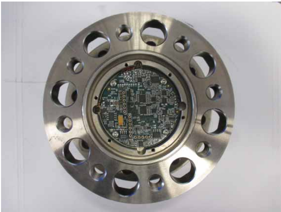
09_DF2 plus Rotor intern
