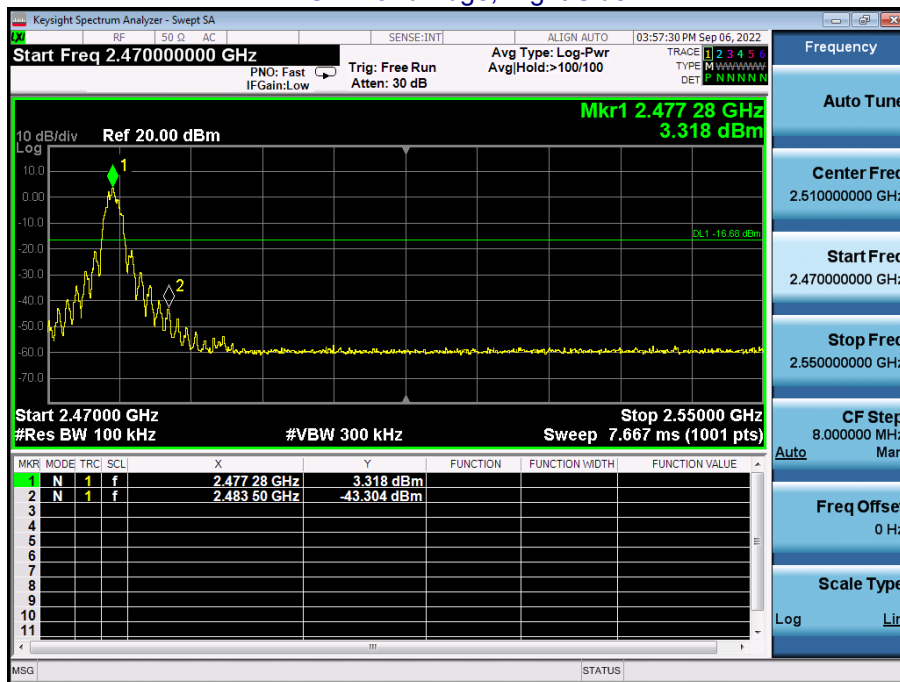
FSK: Band Edge, Right Side
