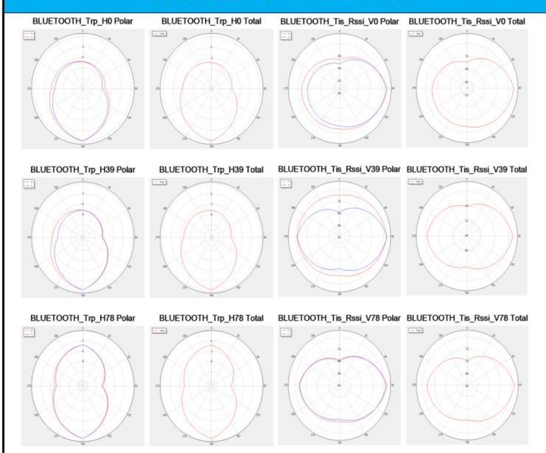
F5-有源方向图- (L自由空间)
