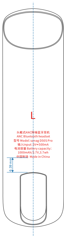
L内侧丝印示意图
