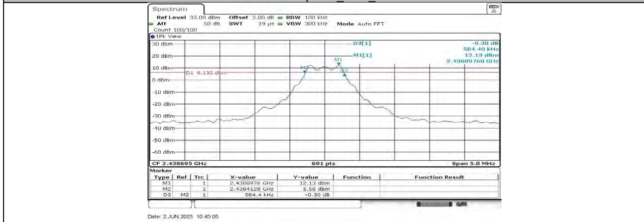
2GFSK-400 kbps.LP_Ant1_MCH
