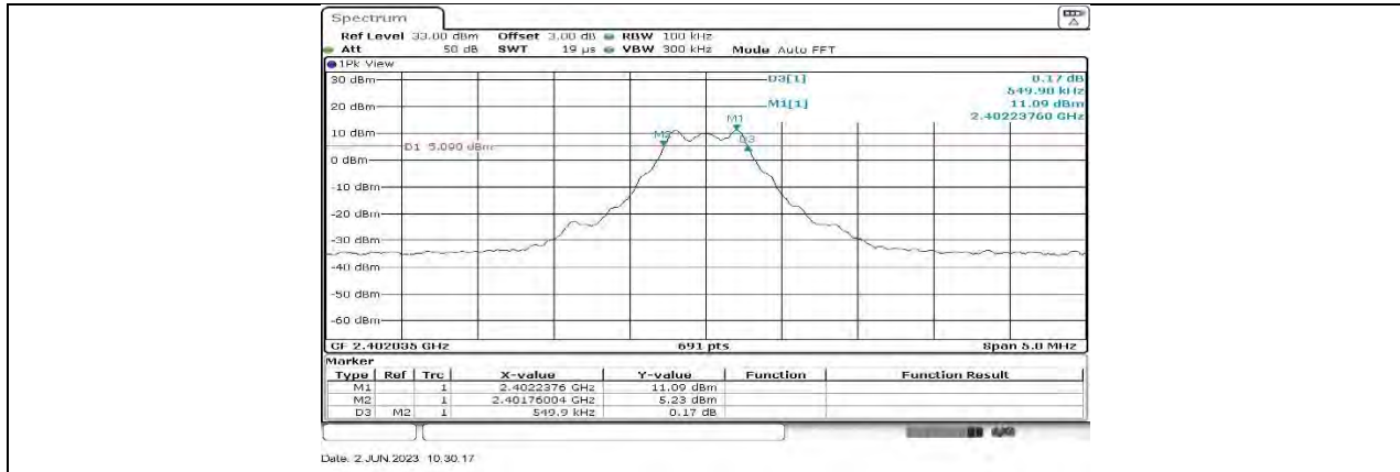
2GFSK-400 kbps.LP_Ant1_LCH.035
