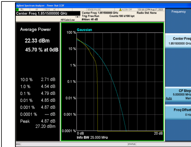
Band2-3MHz-QPSK-18615-1RB#0-PASS
