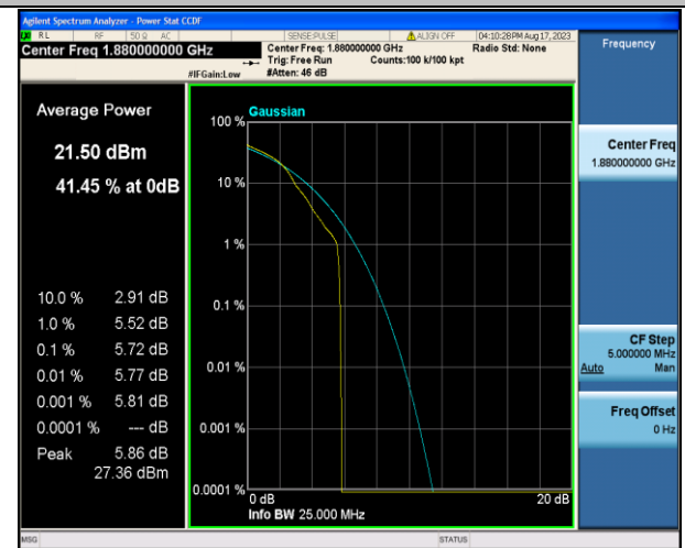
Band2-20MHz-16QAM-18900-1RB#0-PASS
