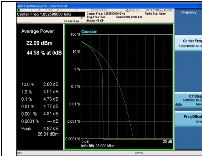
Band2-5MHz-QPSK-18625-1RB#0-PASS
