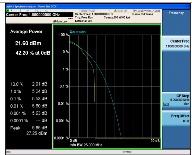
Band2-20MHz-16QAM-18700-1RB#0-PASS
