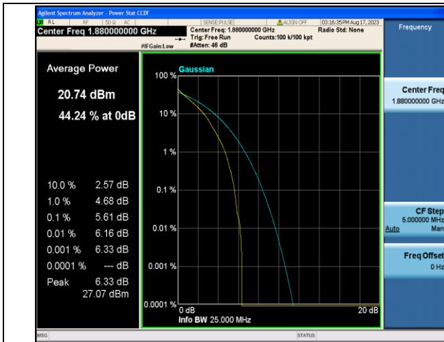
Band2-3MHz-QPSK-18900-15RB#0-PASS
