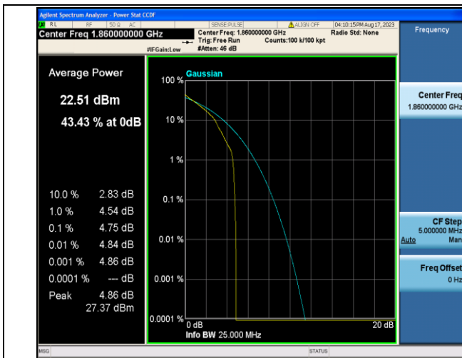
Band2-20MHz-QPSK-18700-1RB#0-PASS
