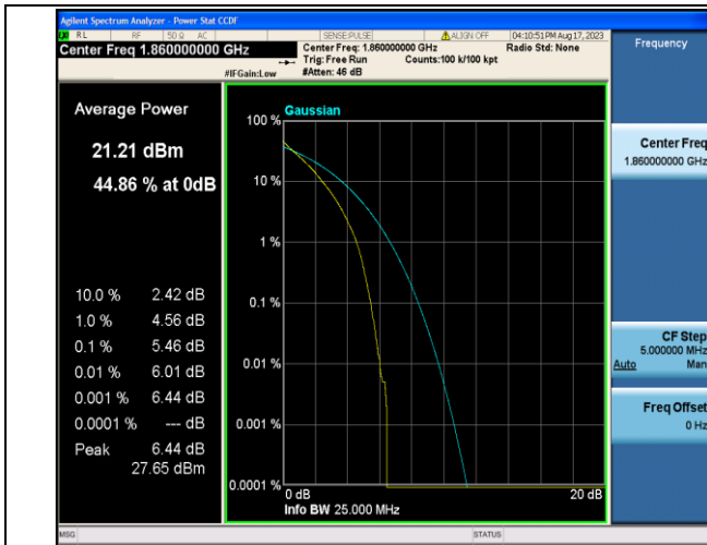
Band2-20MHz-QPSK-18700-100RB#0-PASS
