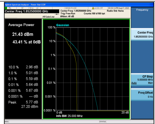
Band2-5MHz-16QAM-18625-1RB#0-PASS
