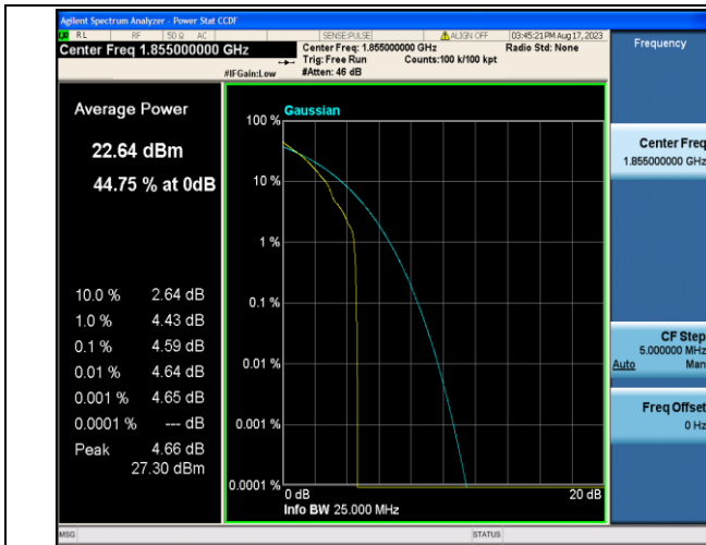
Band2-10MHz-QPSK-18650-1RB#0-PASS
