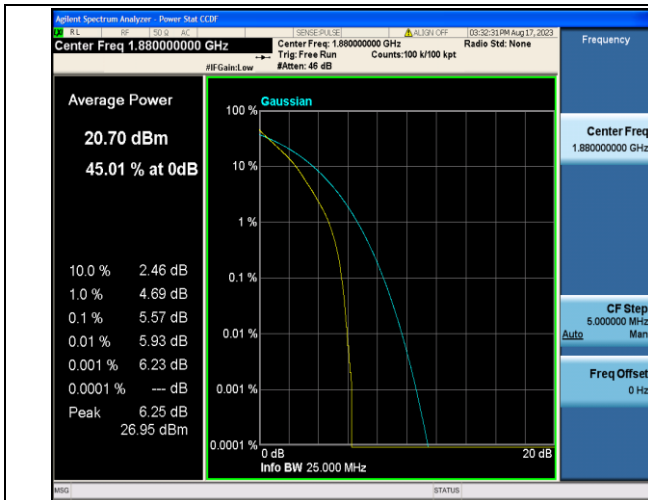
Band2-5MHz-QPSK-18900-25RB#0-PASS
