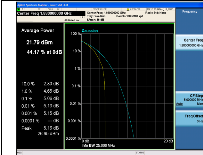
Band2-3MHz-QPSK-18900-1RB#0-PASS
