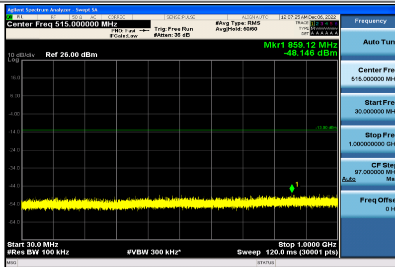
Band25-20MHz-QPSK-26140-1RB#0-30~1000MHz
