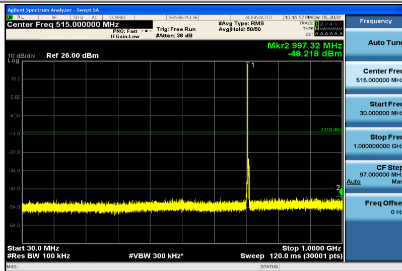
Band12-3MHz-QPSK-23165-1RB#0-30~1000MHz
