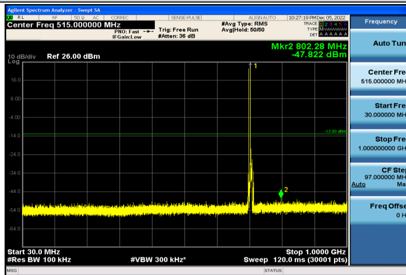
Band12-5MHz-QPSK-23155-1RB#0-30~1000MHz
