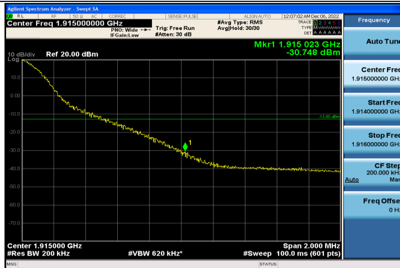
Band25-20MHz-QPSK-26590-1RB#99
