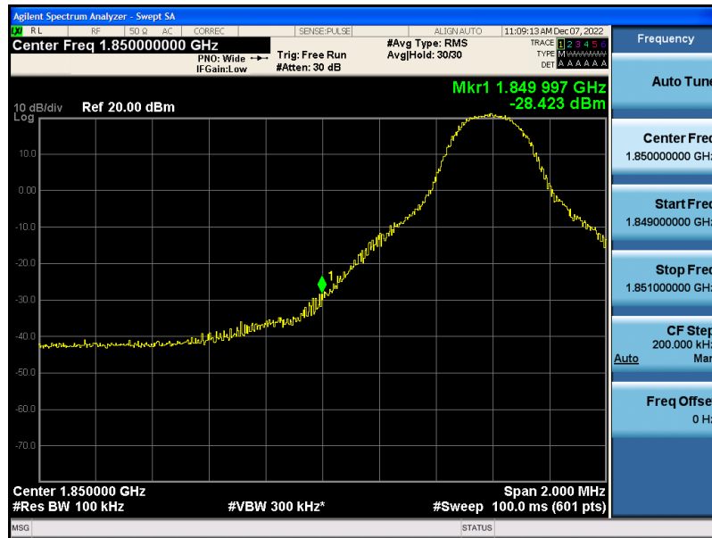
Band2-10MHz-QPSK-18650-1RB#0
