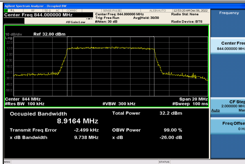
Band26-10MHz-QPSK-26990-50RB#0-8.9164
