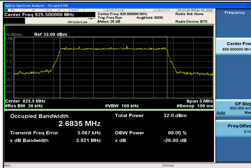
Band5-3MHz-QPSK-20415-15RB#0-2.6835
