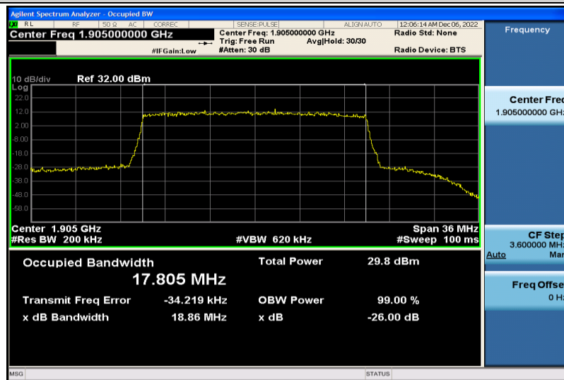
Band25-20MHz-QPSK-26590-100RB#0-17.805
