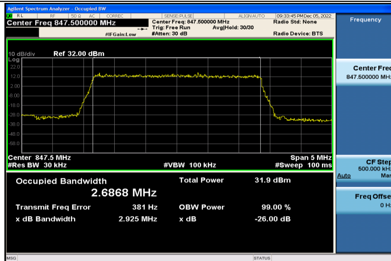
Band5-3MHz-QPSK-20635-15RB#0-2.6868
