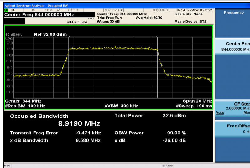
Band5-10MHz-QPSK-20600-50RB#0-8.9190
