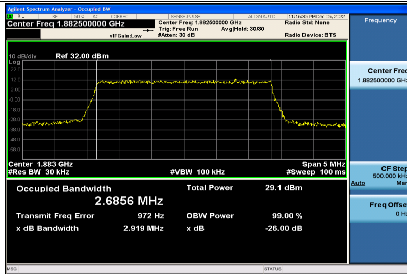
Band25-3MHz-QPSK-26365-15RB#0-2.6856
