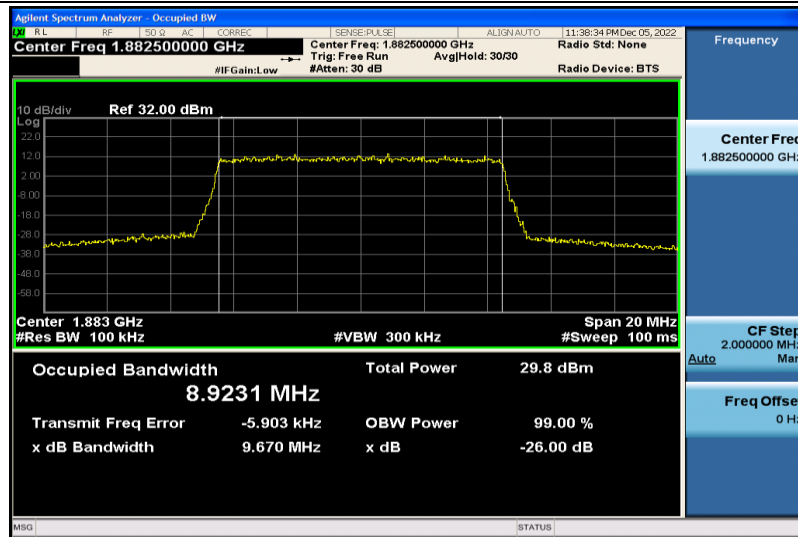
Band25-10MHz-QPSK-26365-50RB#0-8.9231
