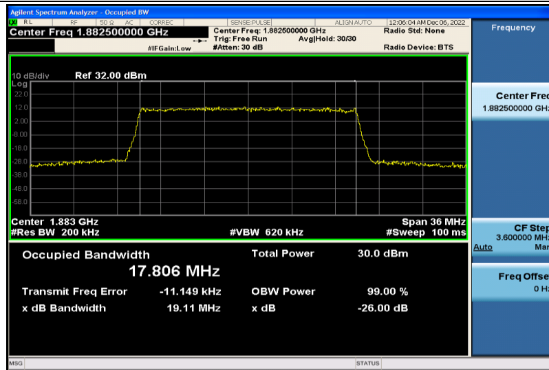
Band25-20MHz-QPSK-26365-100RB#0-17.806
