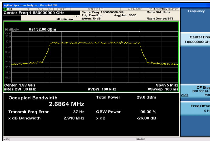
Band2-3MHz-QPSK-18900-15RB#0-2.6864
