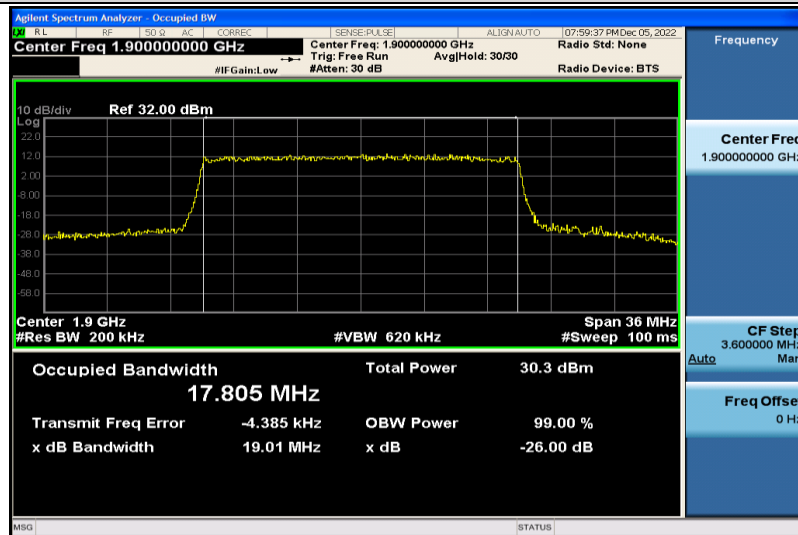
Band2-20MHz-QPSK-19100-100RB#0-17.805
