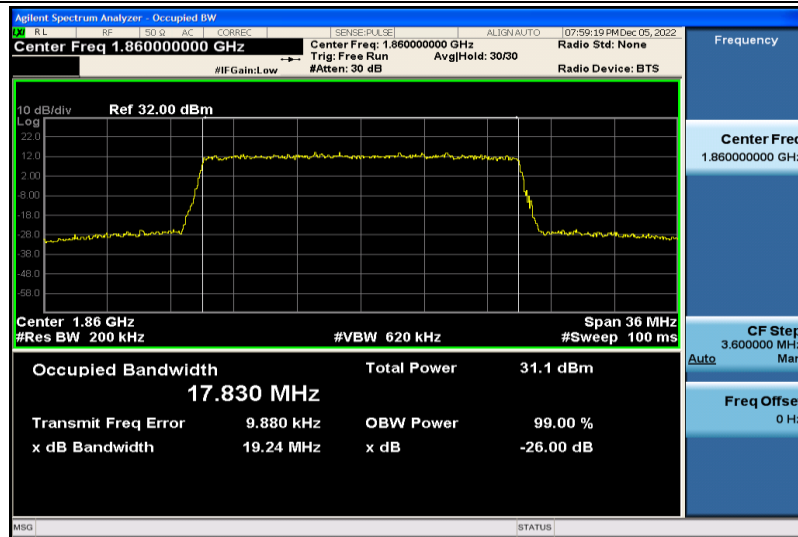
Band2-20MHz-QPSK-18700-100RB#0-17.830
