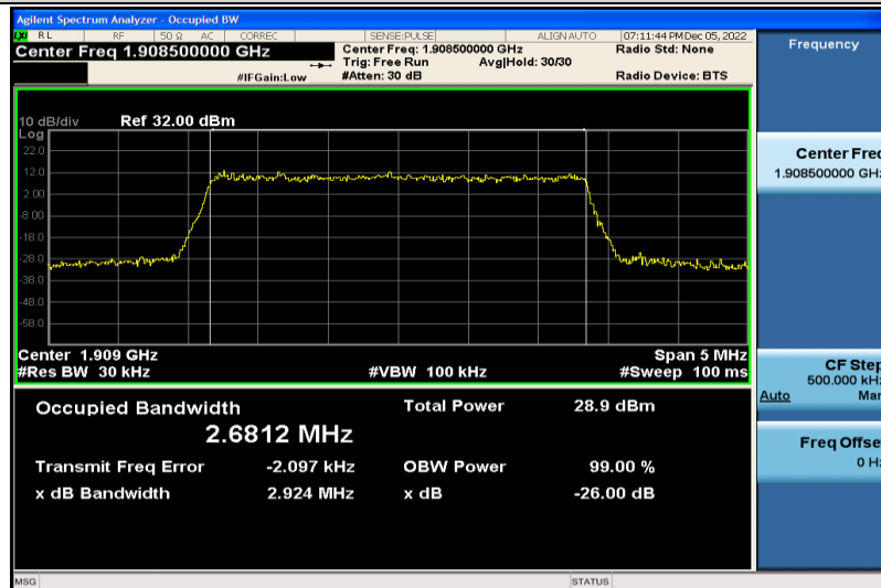
Band2-3MHz-QPSK-19185-15RB#0-2.6812
