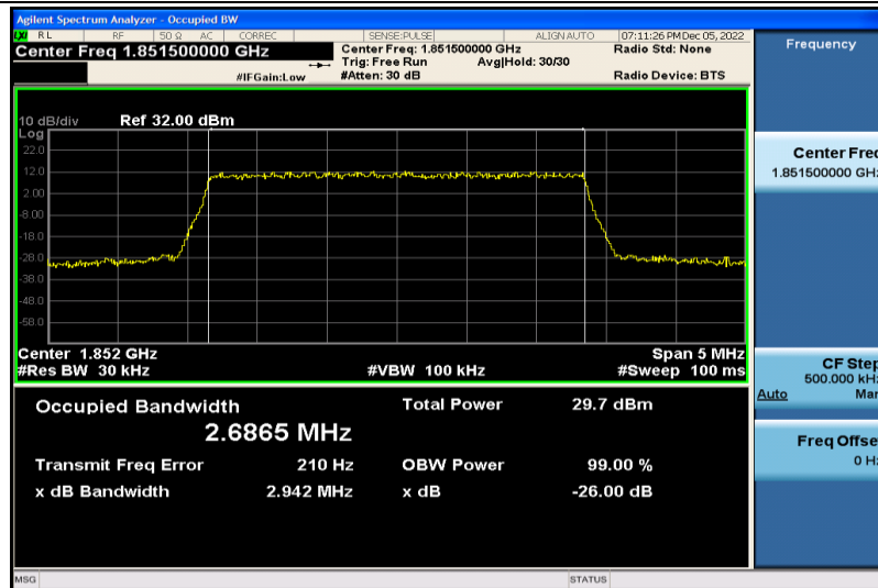
Band2-3MHz-QPSK-18615-15RB#0-2.6865
