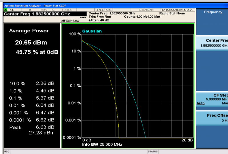
Band25-20MHz-QPSK-26365-100RB#0
