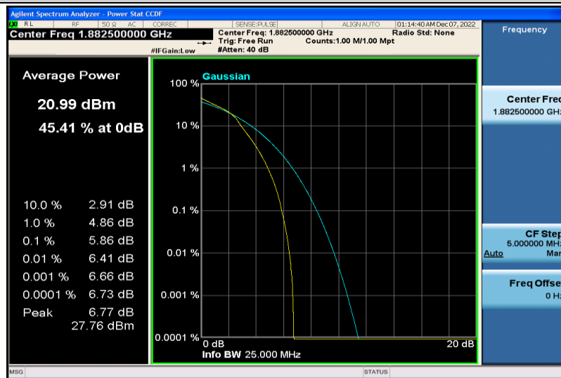
Band25-20MHz-16QAM-26365-25RB#0
