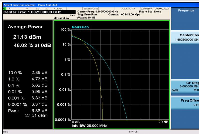
Band25-10MHz-16QAM-26365-25RB#0
