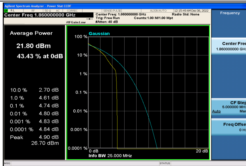
Band25-20MHz-QPSK-26140-1RB#0
