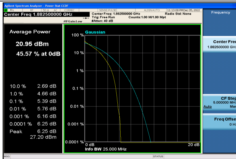
Band25-1.4MHz-QPSK-26365-6RB#0
