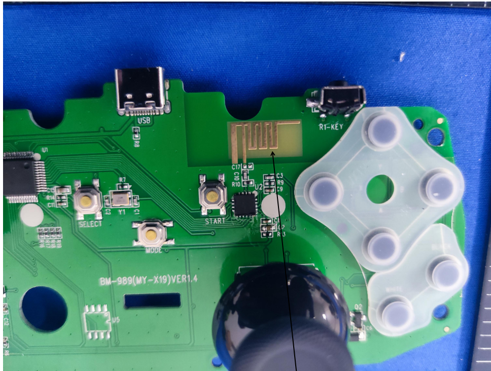
PCB ANT
