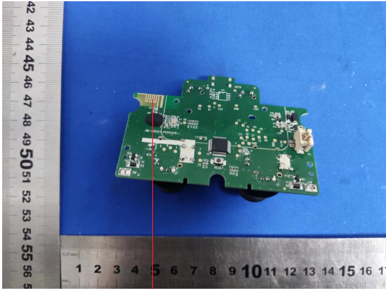
PCB ANT
