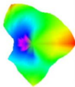
2450.000MHz
