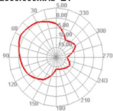
2500.000MHz E1
