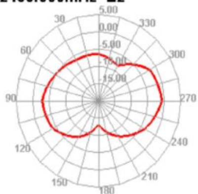
2450.000MHz E2
