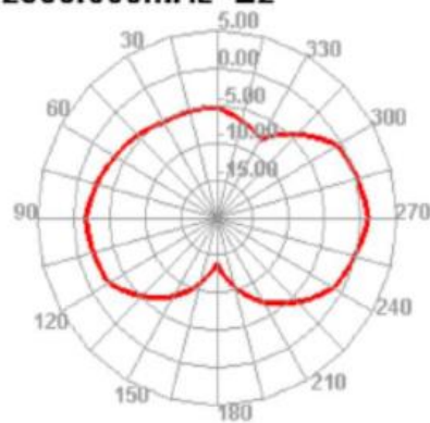
2500.000MHz E2
