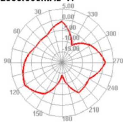
2500.000MHz E2
