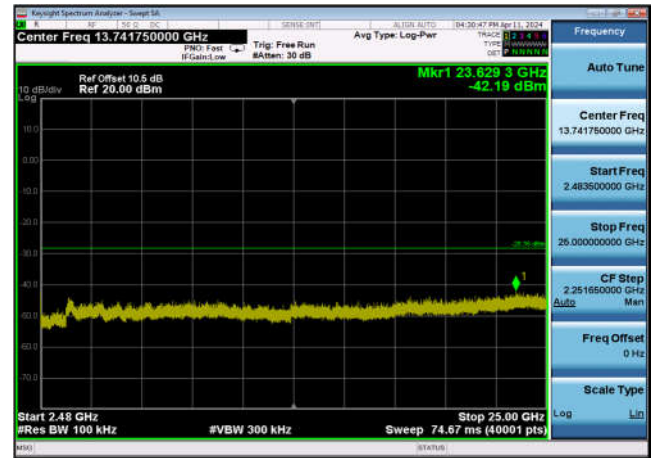
,Plot 4,2483.5MHz~25000MHz-802.11ax(40MHz),2452MHz,Ant12
