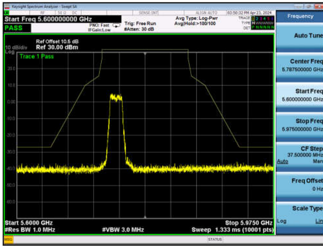
U-NII-3 Band Edge-802.11n(40MHz) ,5755MHz,Ant1
