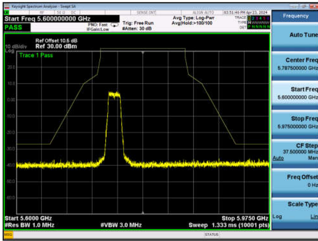
U-NII-3 Band Edge-802.11ac(40MHz) ,5755MHz,Ant1
