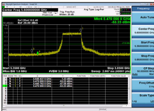
U-NII-2c Band Edge-802.11ac(80MHz) ,5610MHz,Ant1
