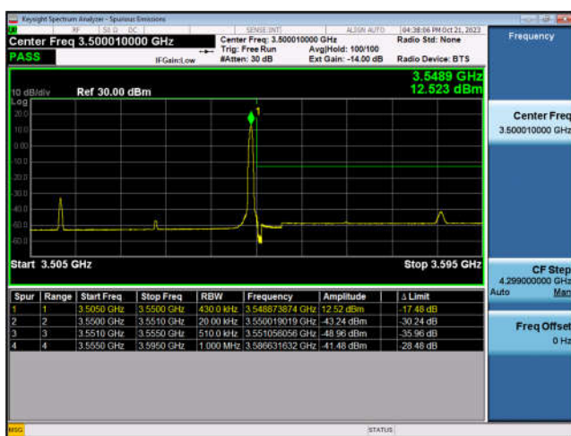
N78_60MHz_DFT-s-OFDM_PI/2-BPSK_Edge_1RB_Left_Low_CH
