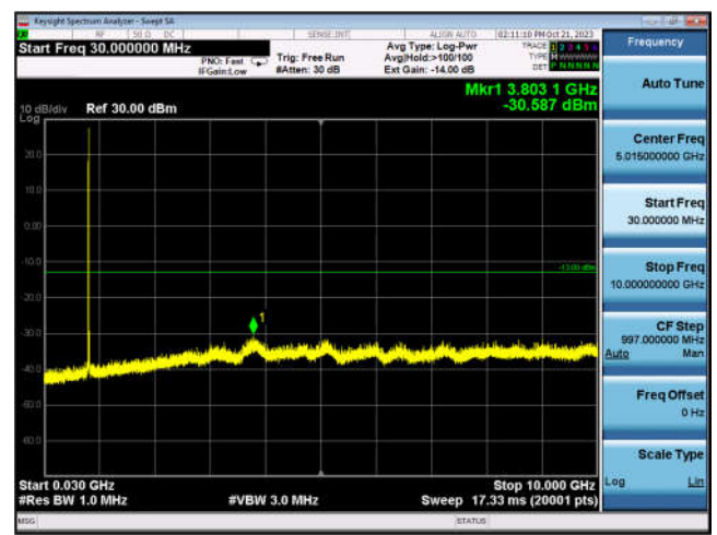
N41_100MHz_DFT-s-OFDM_BPSK_ Edge_1RB_Left_Low_CH
