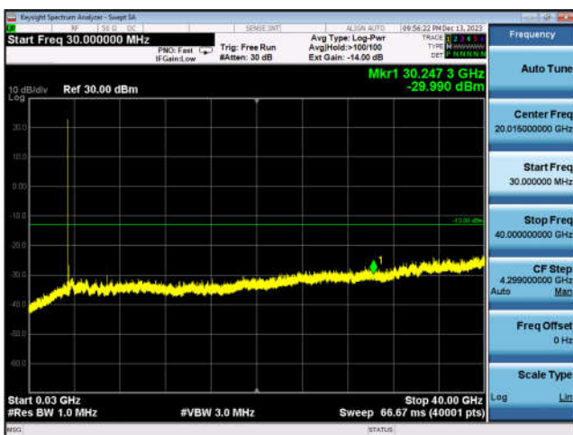
N78_80MHz_DFT-s-OFDM_BPSK_ Edge_1RB_Left_Low_CH
