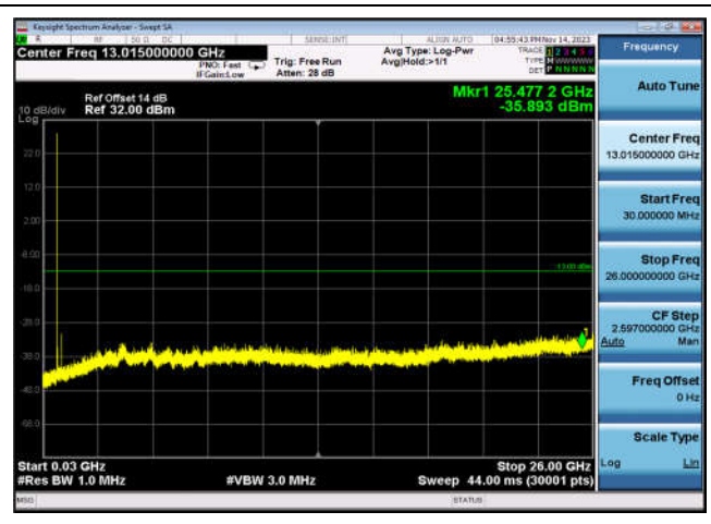
FDD17_HighRange_10MHz_30MHz~26GHz
