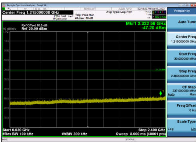
,Plot 3,30MHz~2400MHz-802.11ax(HT20) ,2462MHz,Ant7
