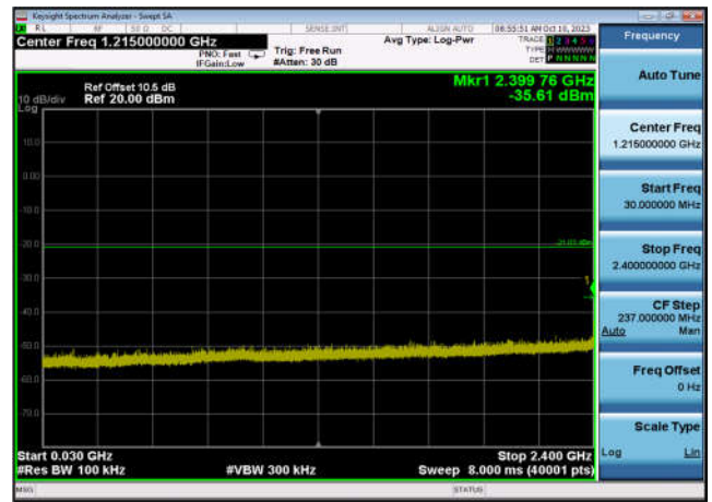
,Plot 3,30MHz~2400MHz-802.11ax(HT20) ,2437MHz,Ant9
