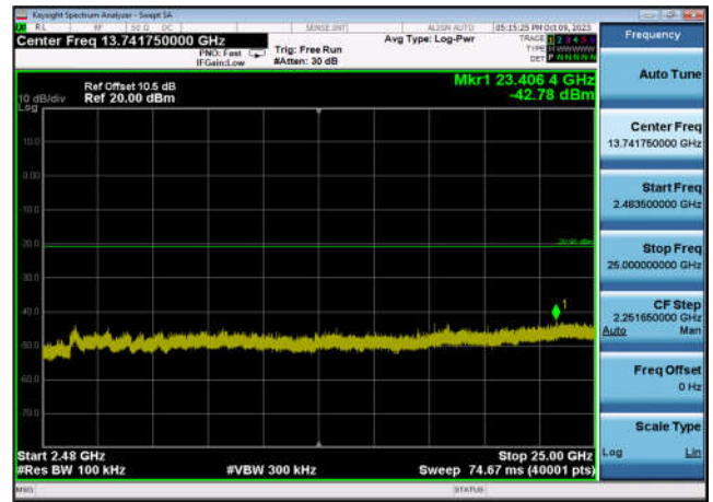
,Plot 4,2483.5MHz~25000MHz-802.11n(HT 20),2462MHz,Ant9
