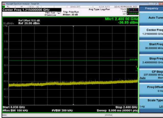
,Plot 3,30MHz~2400MHz-802.11ax(HT40) ,2437MHz,Ant7
