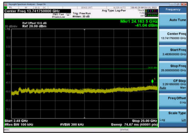
,Plot 4,2483.5MHz~25000MHz-802.11n(HT 40),2437MHz,Ant9
