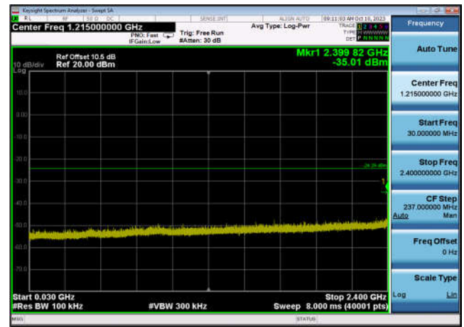
,Plot 3,30MHz~2400MHz-802.11ax(HT40) ,2437MHz,Ant9
