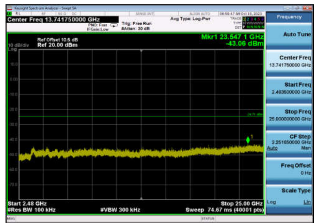
,Plot 4,2483.5MHz~25000MHz-802.11n(HT 40),2452MHz,Ant9
