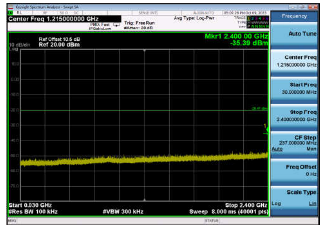
,Plot 3,30MHz~2400MHz-802.11n(HT20) ,2437MHz,Ant9
