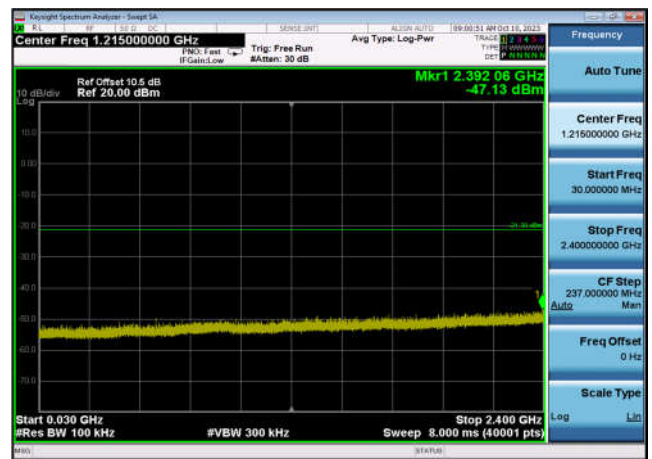
,Plot 3,30MHz~2400MHz-802.11ax(HT20) ,2462MHz,Ant9
