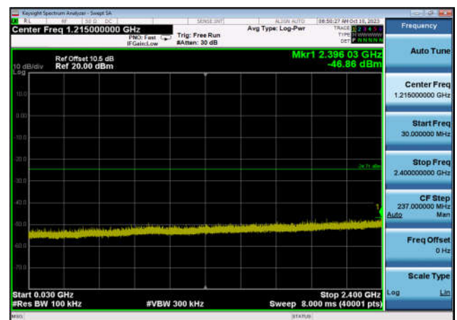
,Plot 3,30MHz~2400MHz-802.11n(HT40) ,2452MHz,Ant9
