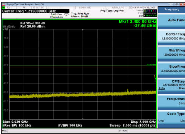
,Plot 3,30MHz~2400MHz-802.11ax(HT20) ,2437MHz,Ant7
