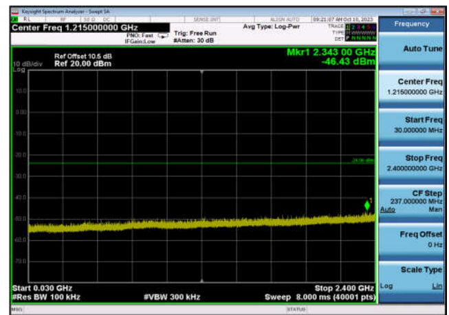
,Plot 3,30MHz~2400MHz-802.11ax(HT40) ,2452MHz,Ant9
