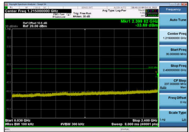
,Plot 3,30MHz~2400MHz-802.11n(HT40) ,2437MHz,Ant9
