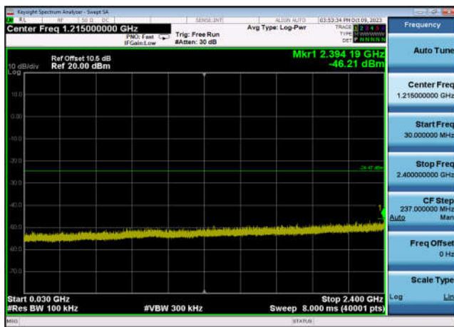
,Plot 3,30MHz~2400MHz-802.11ax(HT40) ,2452MHz,Ant7
