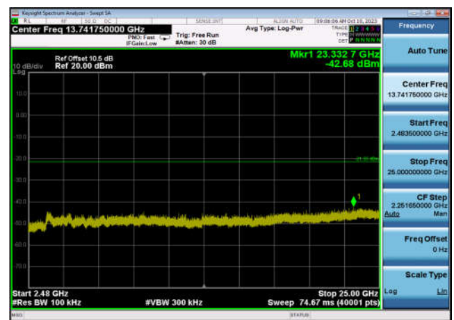
,Plot 4,2483.5MHz~25000MHz-802.11ax(H T20),2462MHz,Ant9
