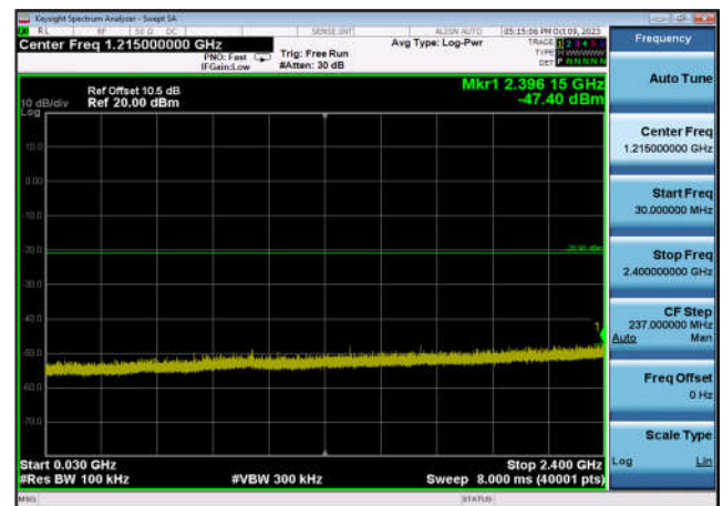
,Plot 3,30MHz~2400MHz-802.11n(HT20) ,2462MHz,Ant9
