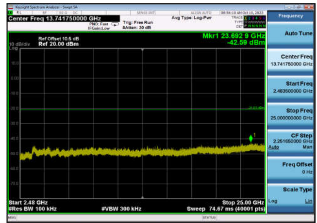
,Plot 4,2483.5MHz~25000MHz-802.11ax(H T20),2437MHz,Ant9
