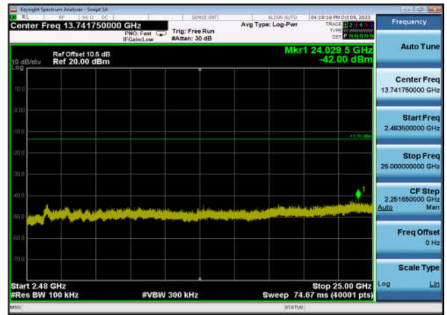
,Plot 4,2483.5MHz~25000MHz-802.11b ,2462MHz,Ant9
