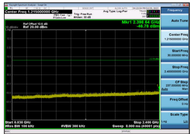
,Plot 3,30MHz~2400MHz-802.11b,2462MHz ,Ant9
