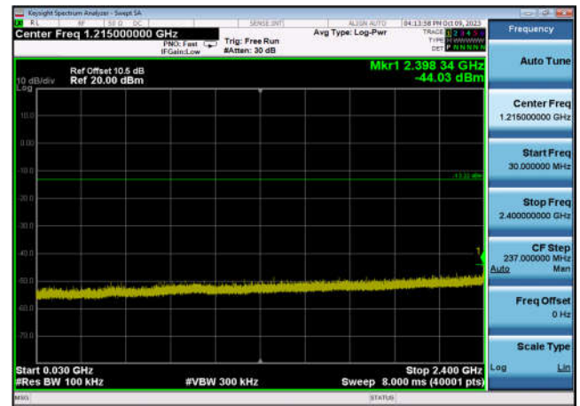
,Plot 3,30MHz~2400MHz-802.11b,2437MHz ,Ant9
