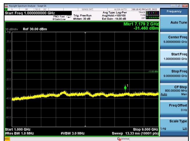
CDMA2000 BC0-777, 1GHz to 9GHz
