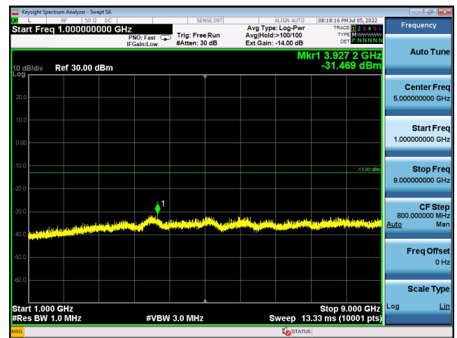
CDMA2000 BC0-777, 1GHz to 9GHz
