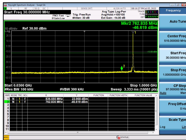
CDMA2000 BC0-777, 30MHz ~1GHz
