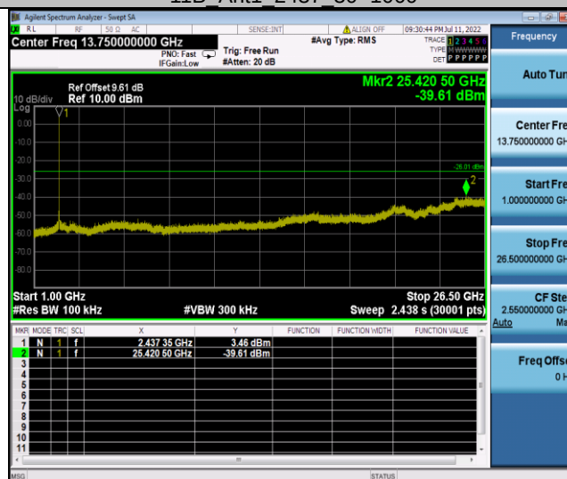
11B_Ant1_2437_1000~26500
