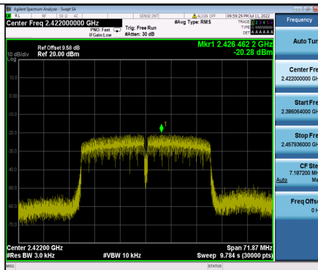
11N40SISO Ant1 2422
