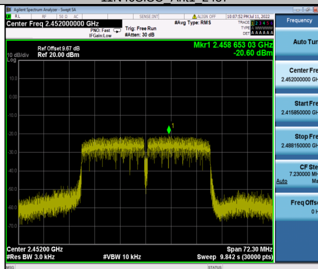
11N40SISO Ant1 2452
