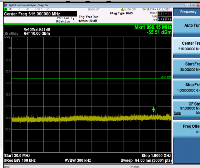
11B_Ant1_2437_30~1000
